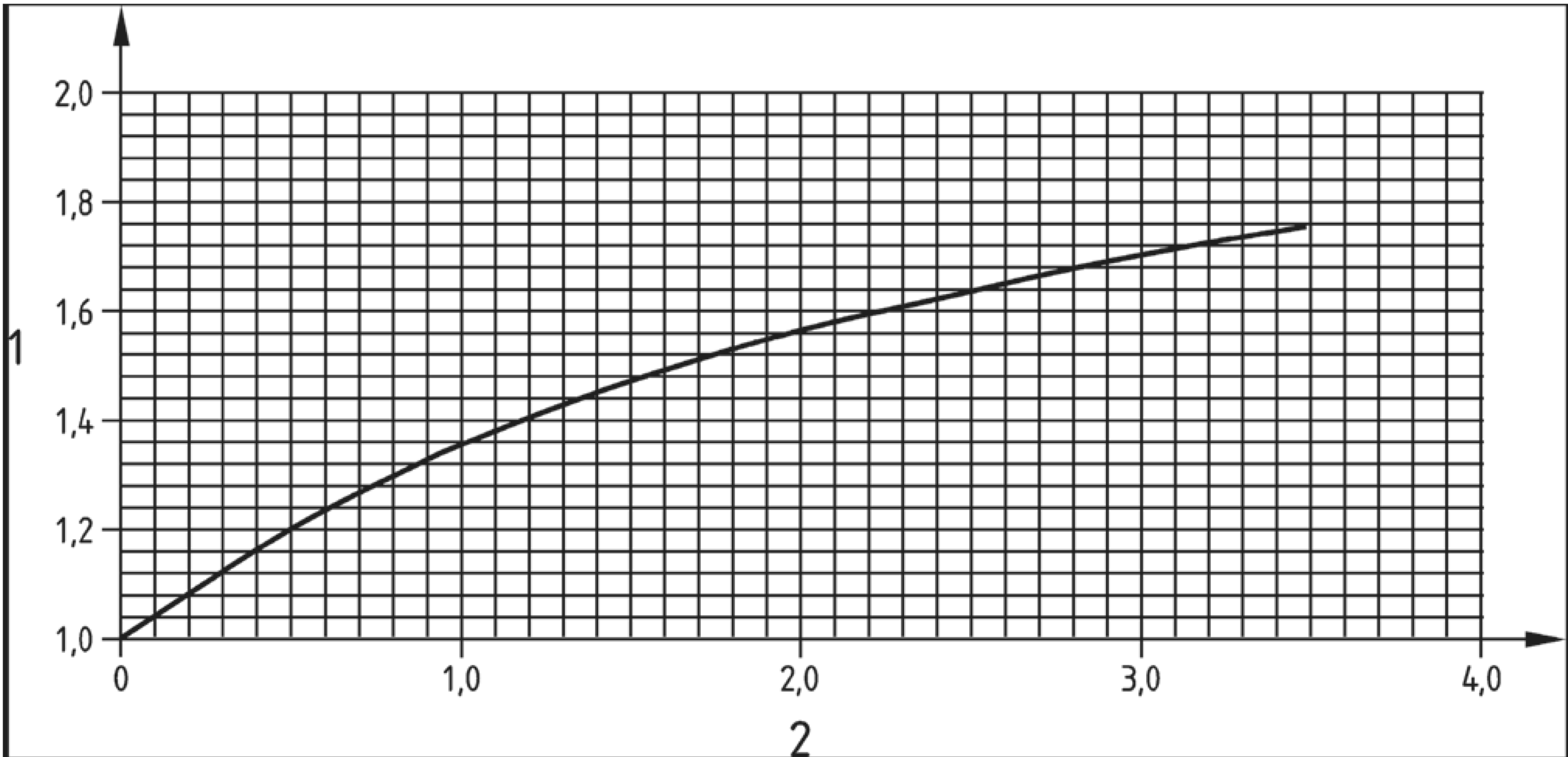
1 – коэффициент \beta 2 – период колебаний T , с
