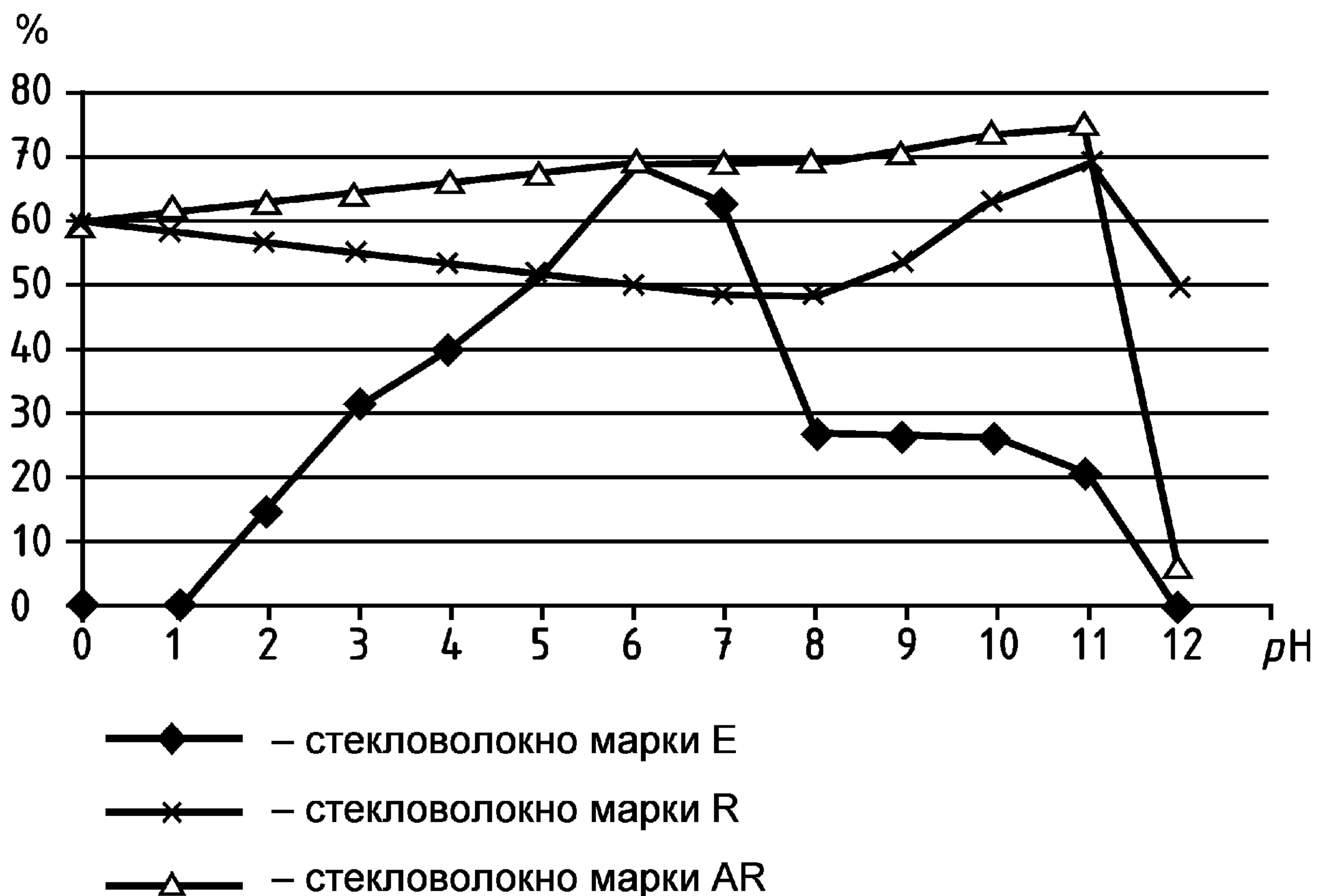
Рисунок А.1 – Коррозионная стойкость стекловолокна различных марок
