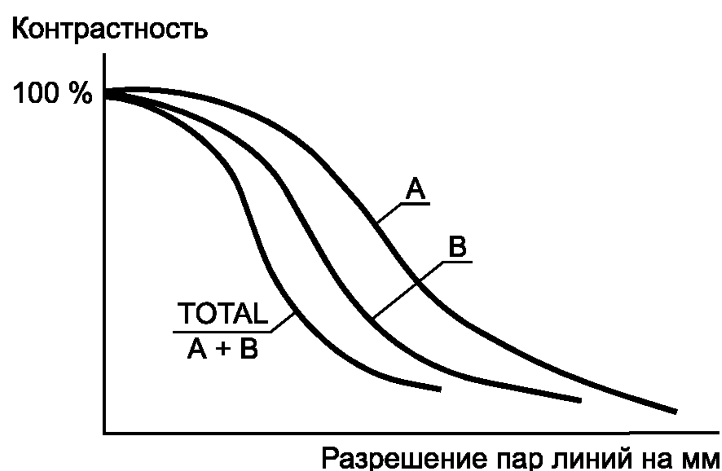
Рисунок ДГ.17 — Типичный график MTF
