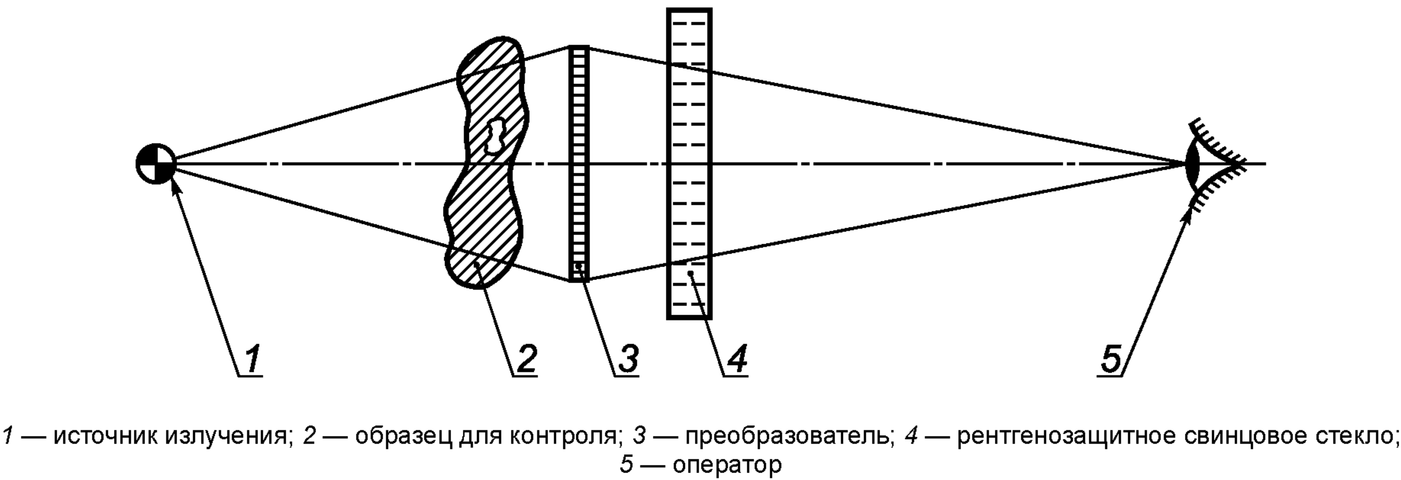
Рисунок ДГ.1 — Основная система радиоскопии
