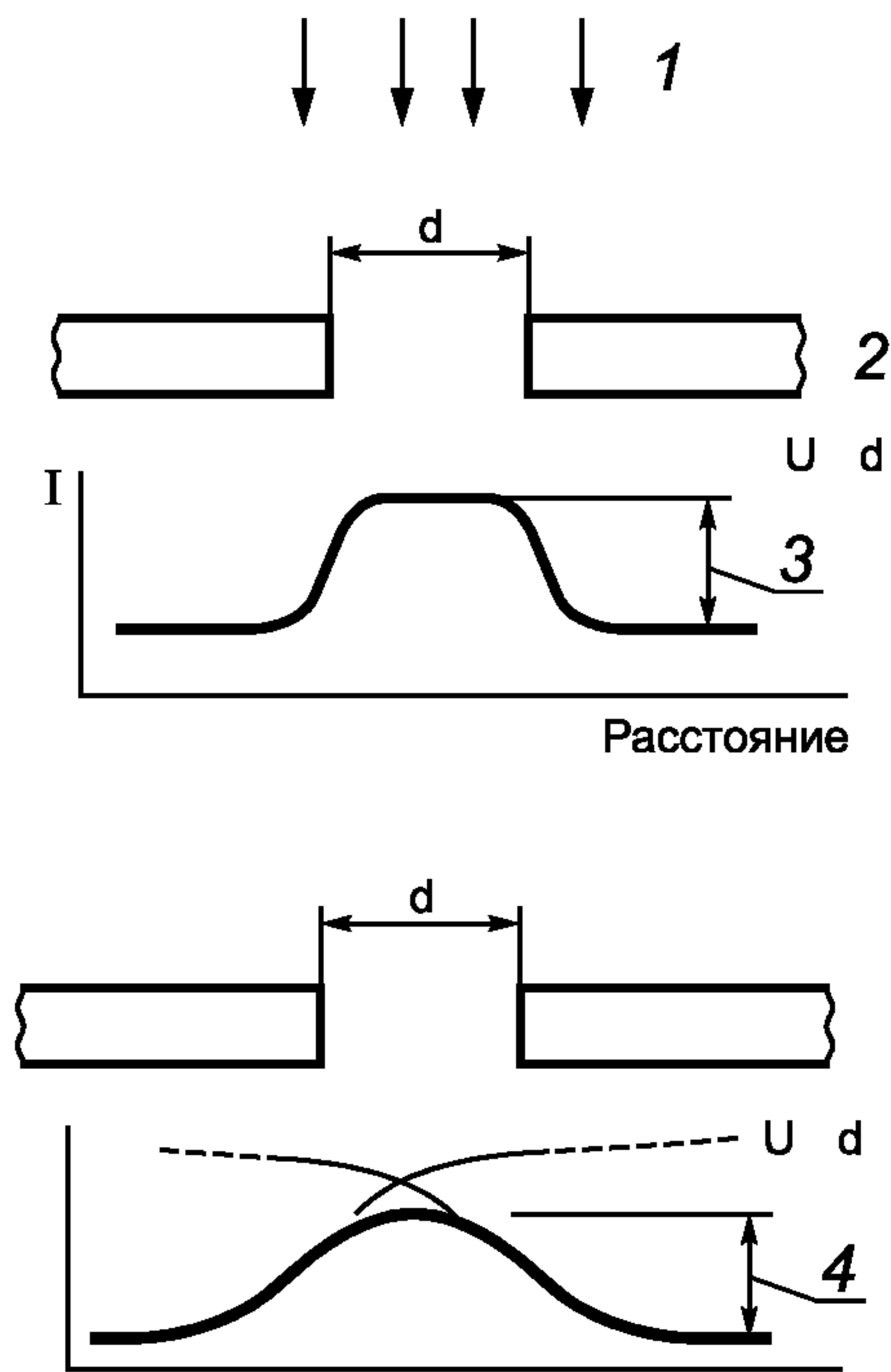
1 — рентгеновские лучи; 2 — образец для контроля; 3 — полная контрастность; 4 — сниженная контрастность
