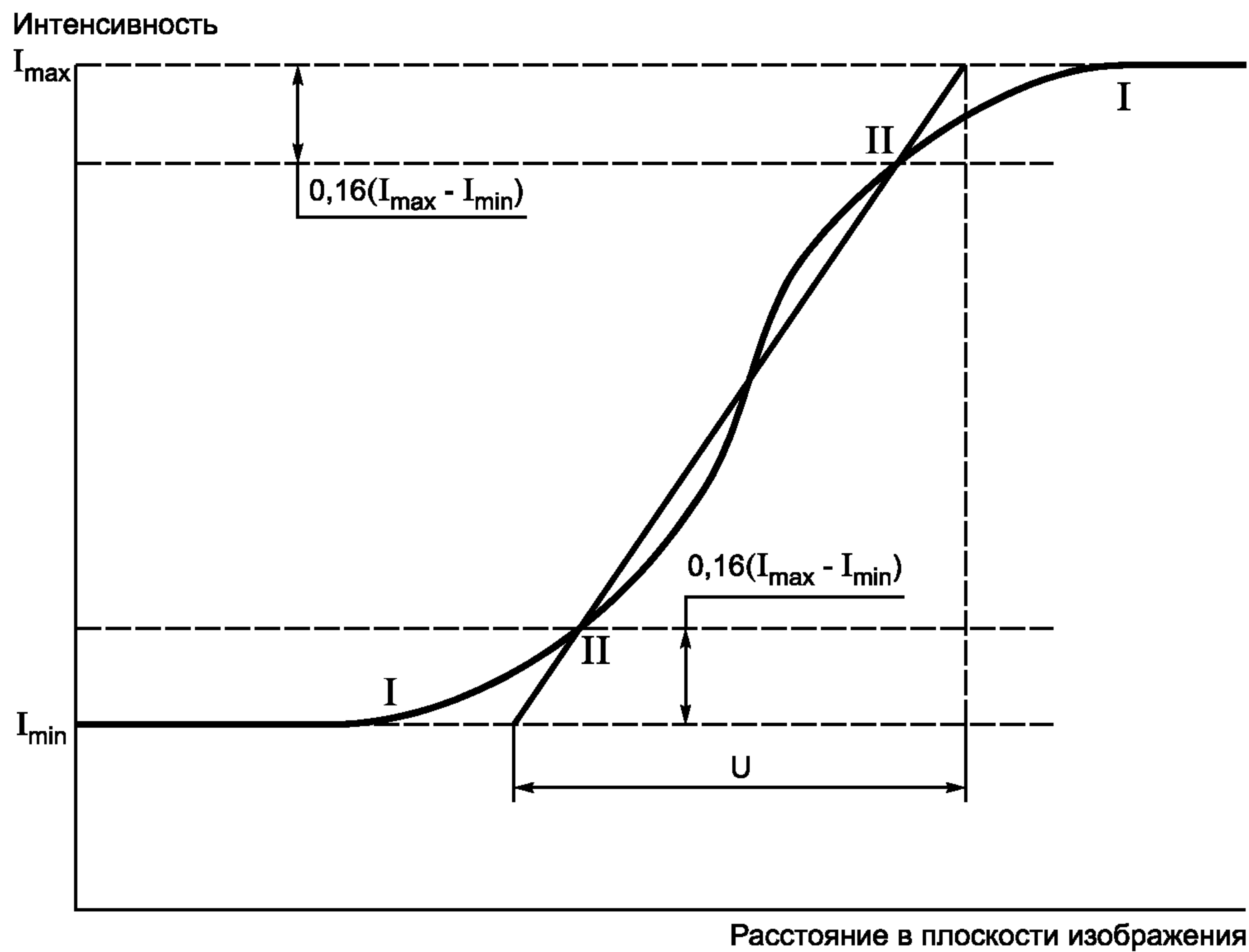
Рисунок ДГ.16 — Метод Классена
