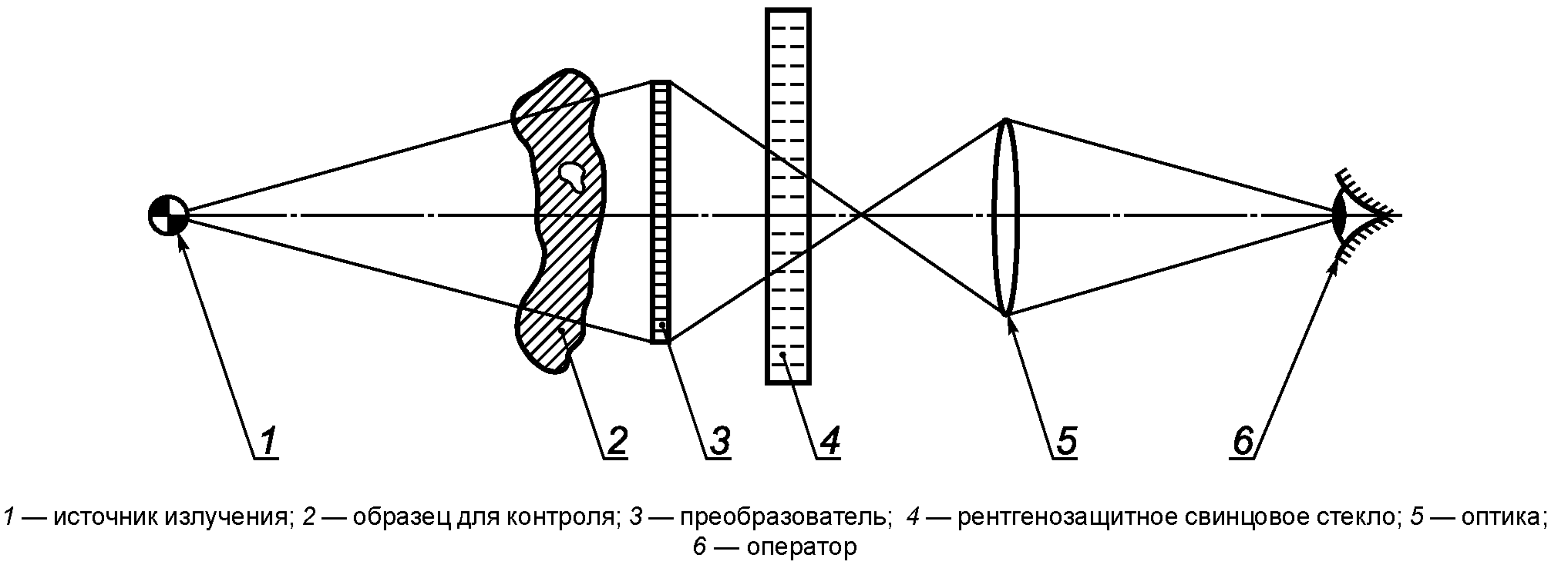
Рисунок ДГ.2 — Система радиоскопии с оптикой
