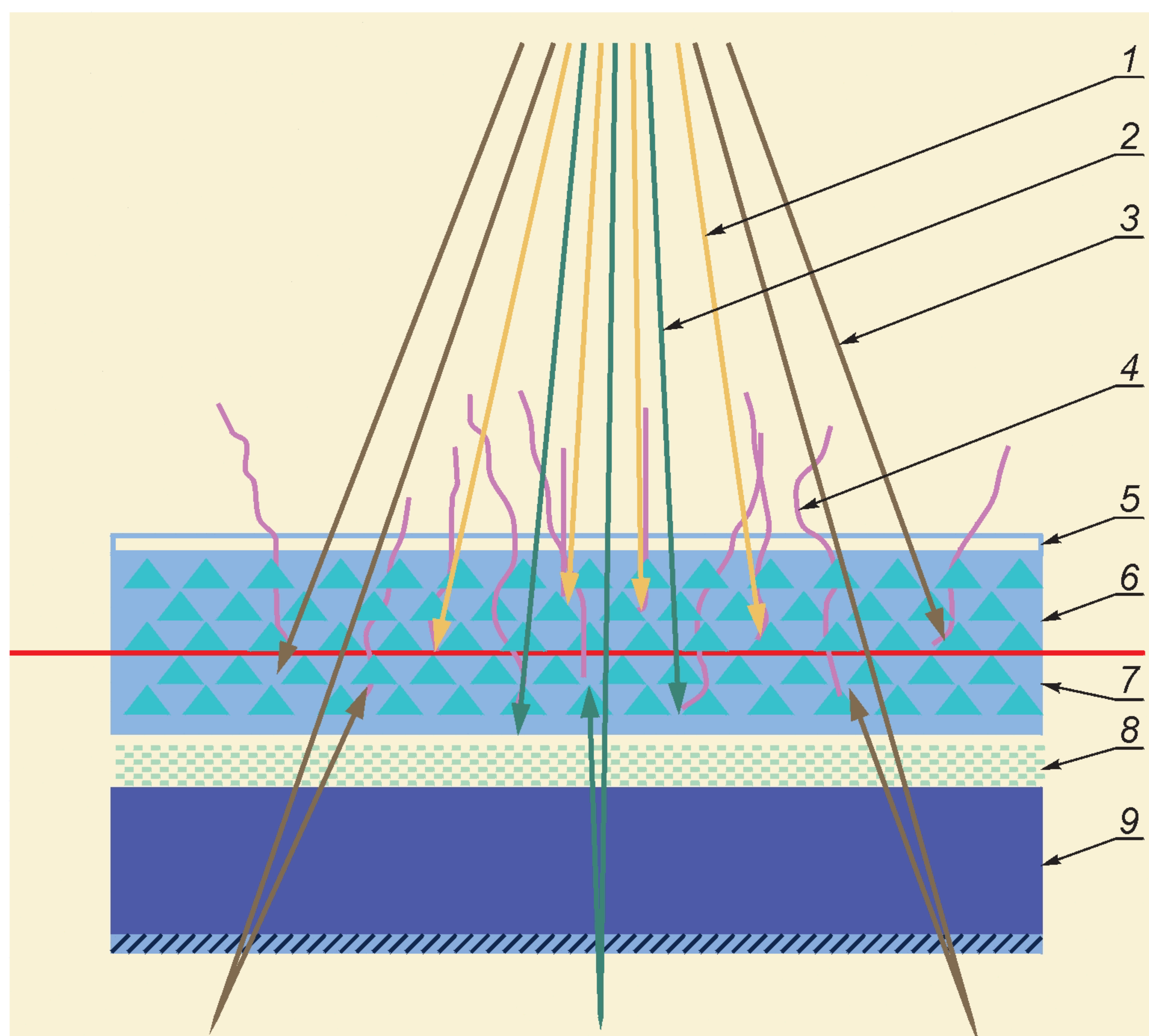
1 — оптимальное излучение; 2 — излучение с высокой энергией; 3 — вторичное с высокой энергией; 4 — ФСЛ; 5 — защитный слой; 6 — верхний люминофорный слой; 7 — нижний люминофорный слой; 8 — проводящий слой; 9 — гибкая подложка
