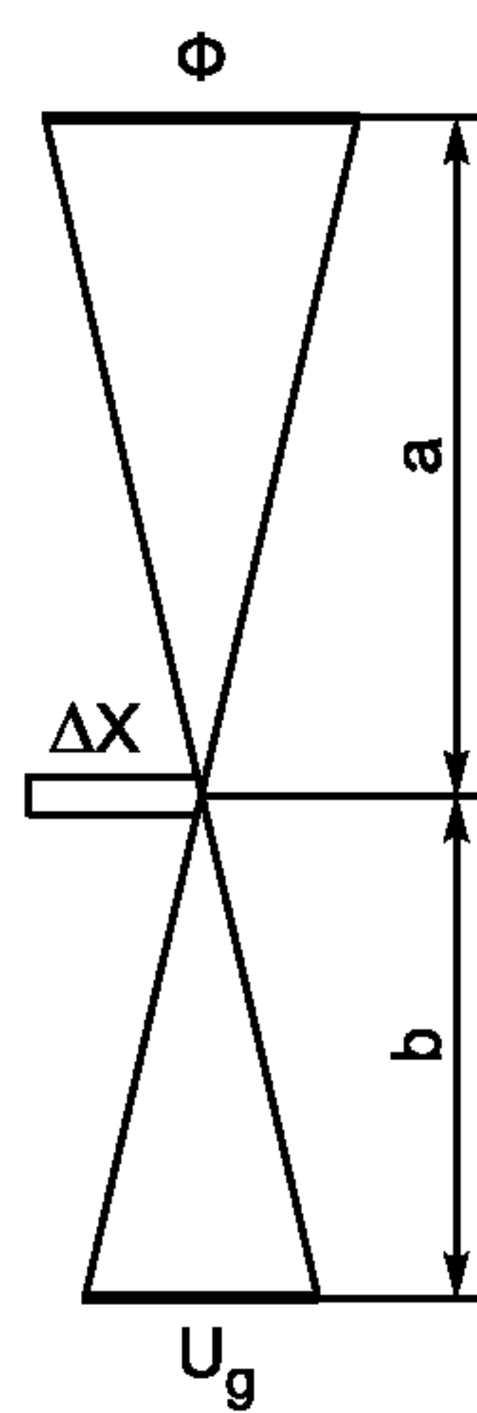
б) Нерезкость, вызванная геометрическими параметрами U_g
