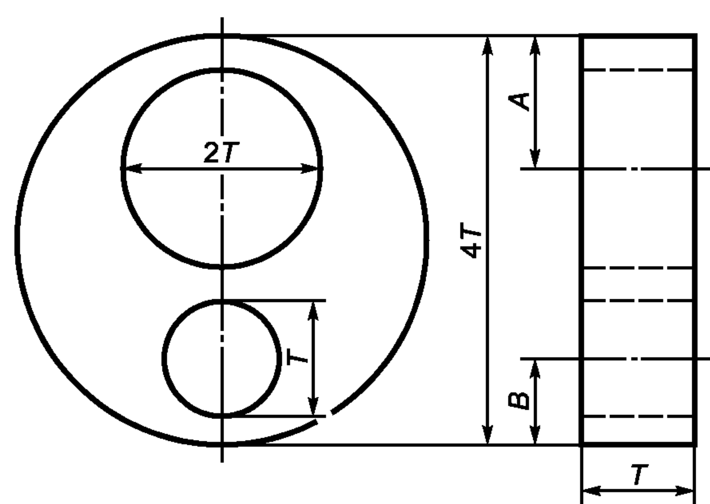
Рисунок 2 — Круглый эталон чувствительности
