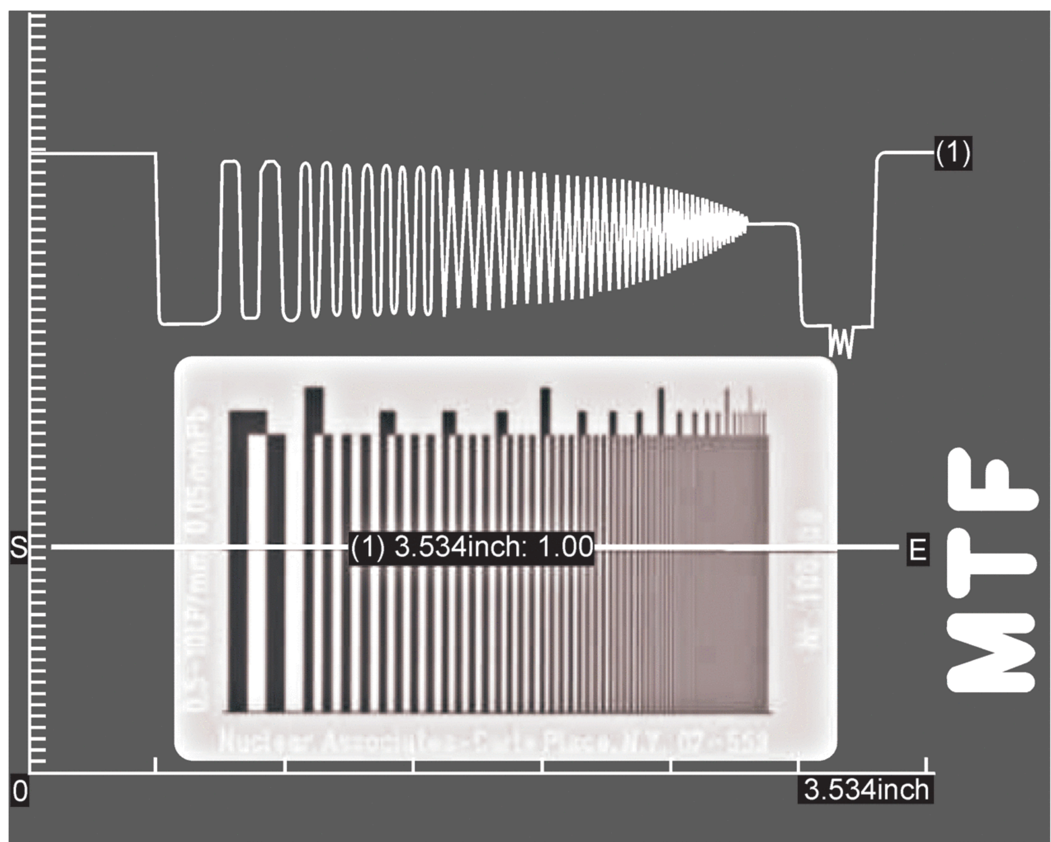
Рисунок ДЕ.6 — Определение разрешения систем формирования изображений
