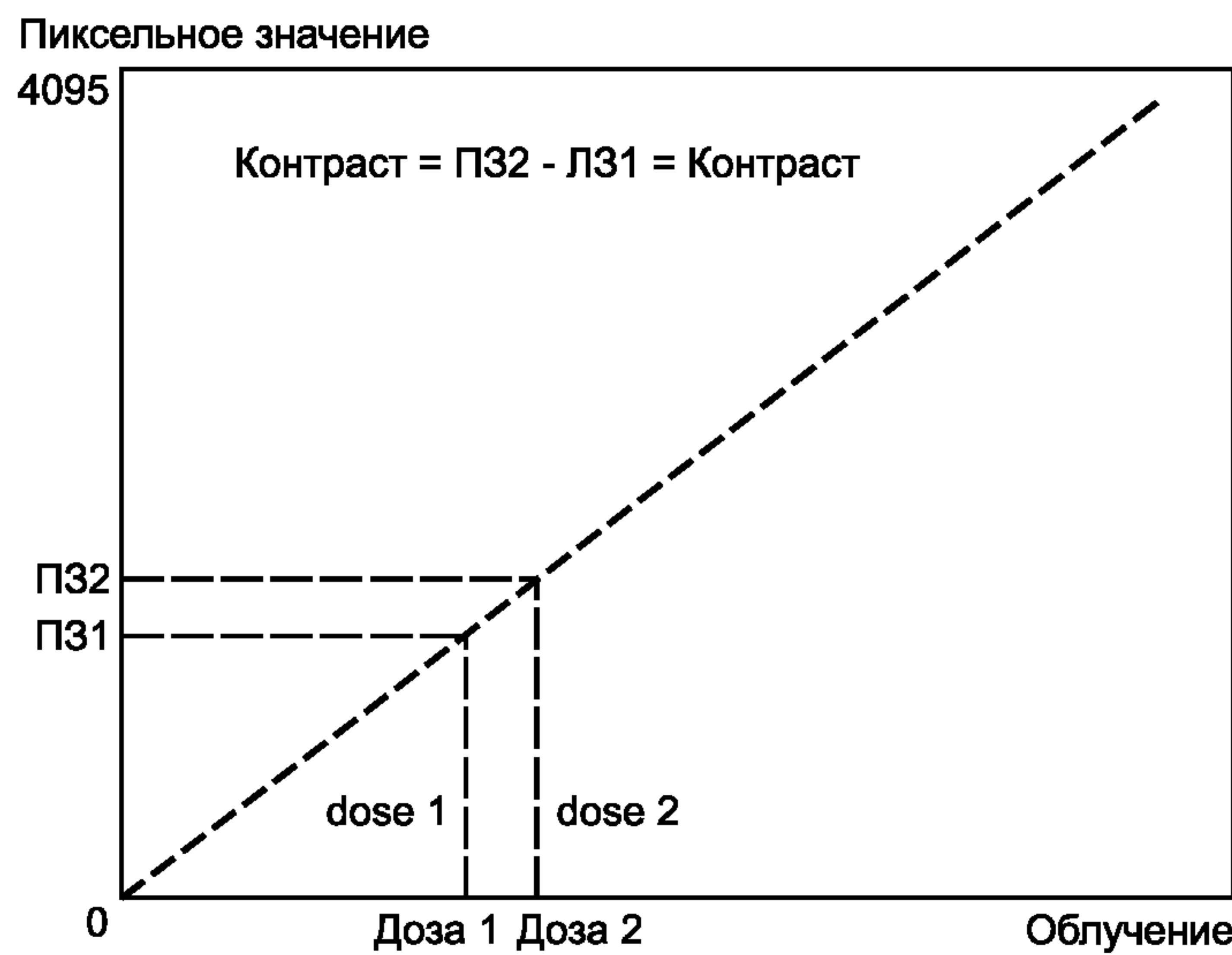
Рисунок ДЕ.3 — Зависимость облучения от пиксельного значения
