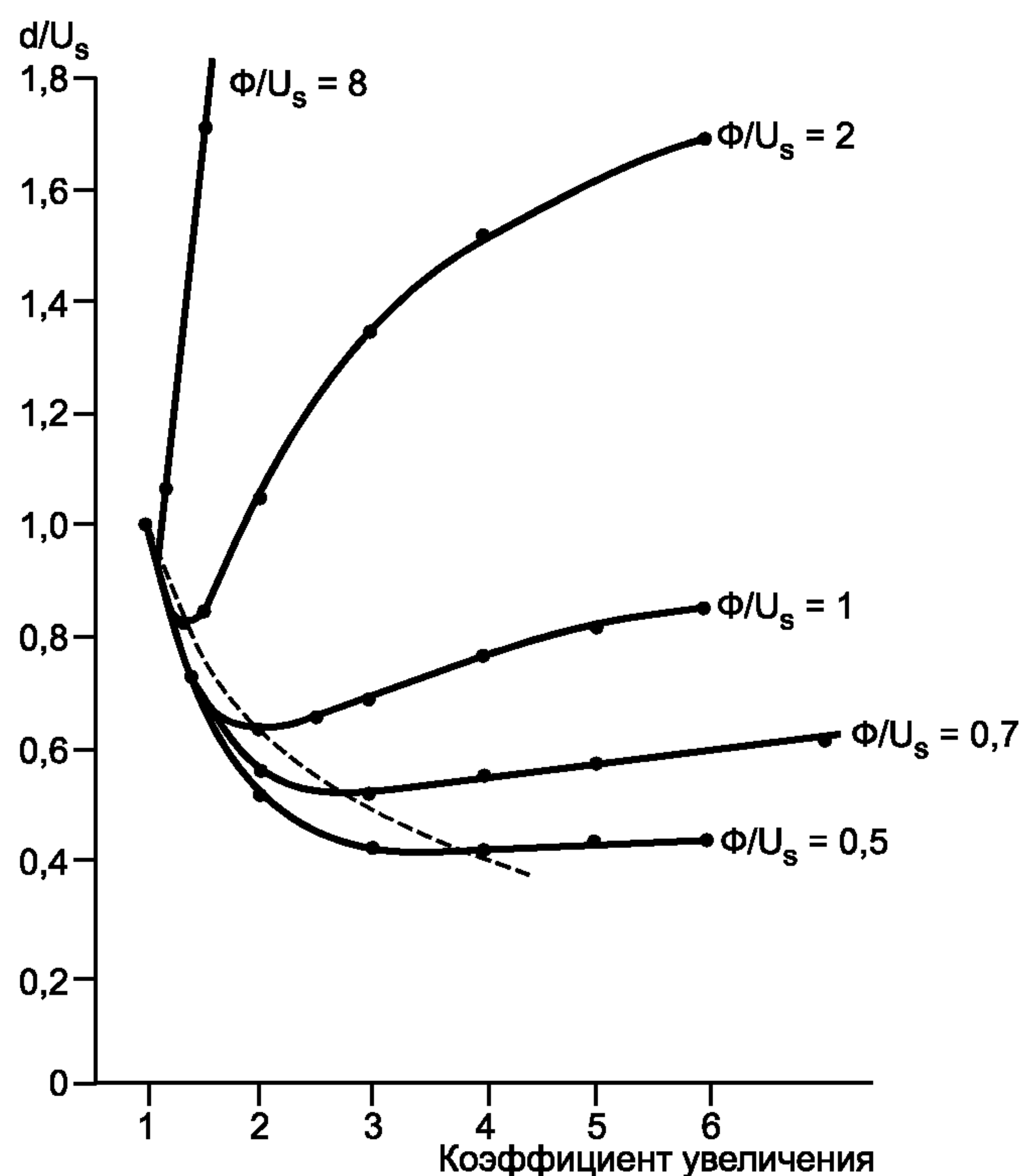
Рисунок ДГ.19 — График дефектов
