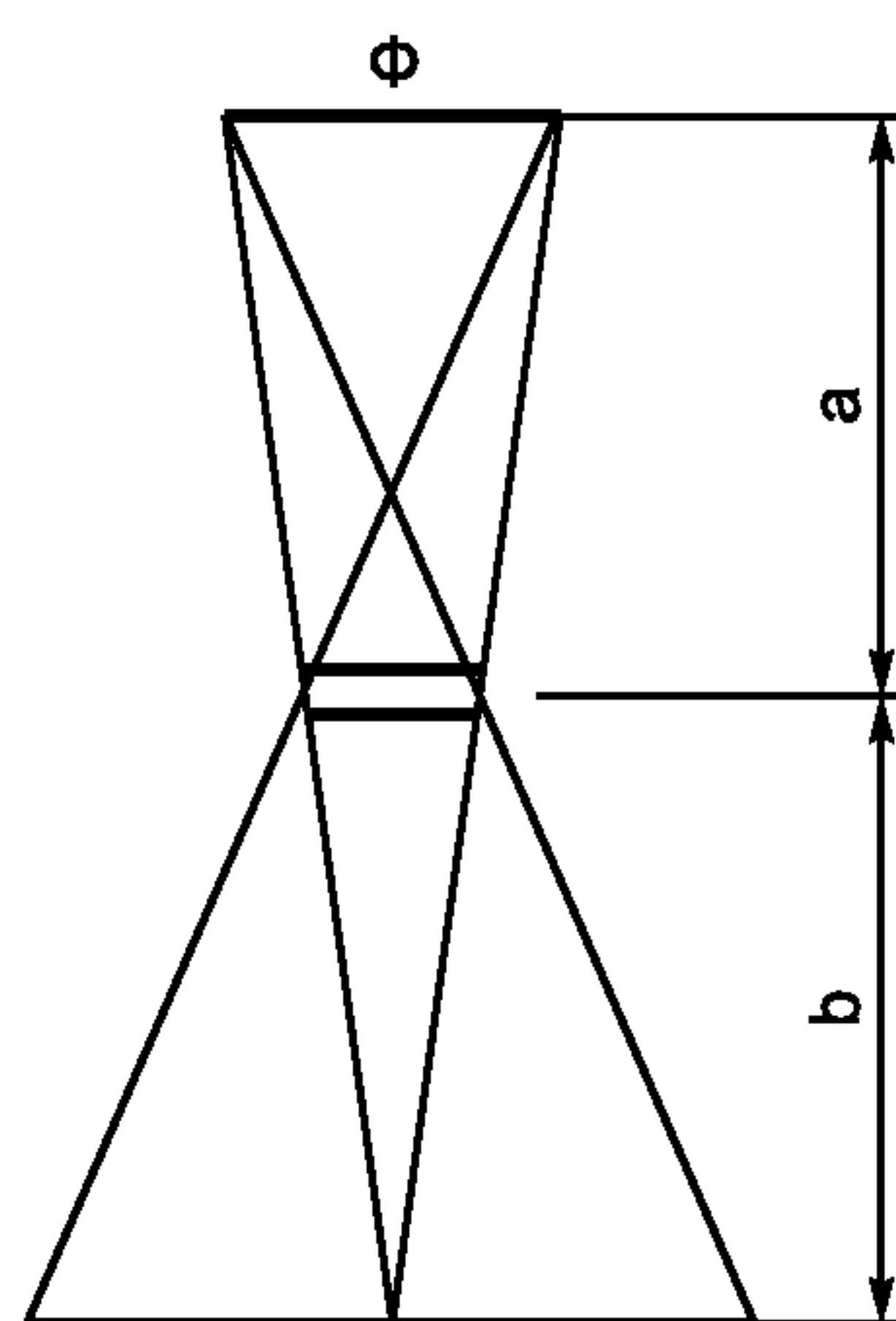
б) Нерезкость, вызванная геометрическими параметрами U_g
