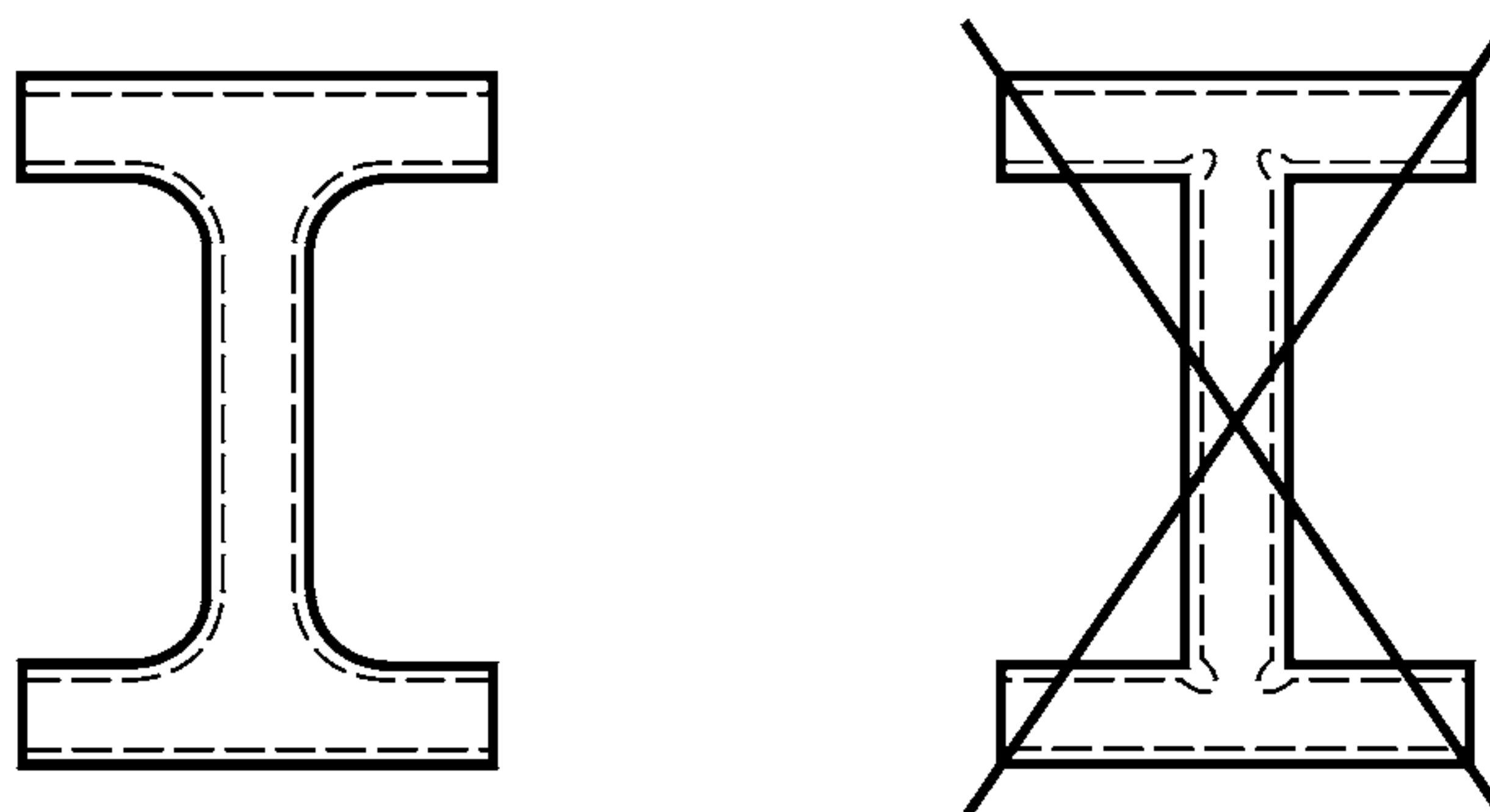
Рисунок Г.3 — Расположение мата в сечении
