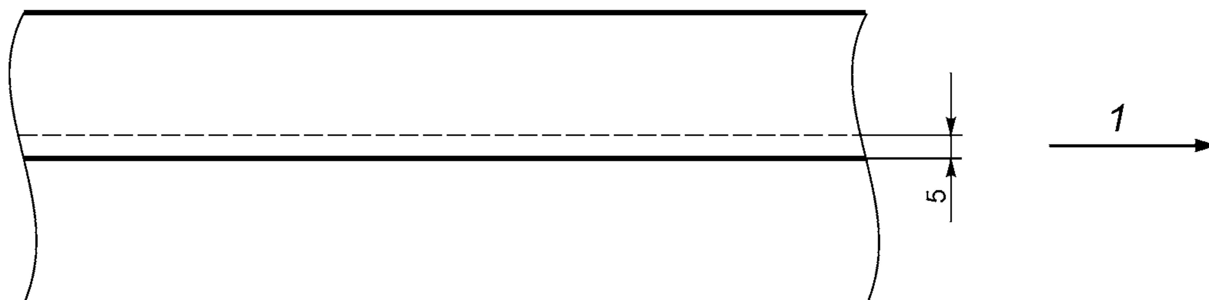
Рисунок Г.1 — Продольные перекрытия мата
