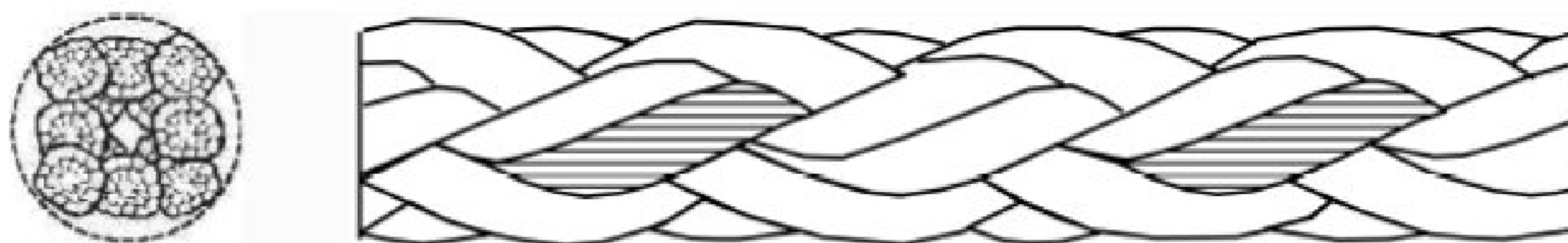
Рисунок 1 — Конфигурация 8-рядного плетеного каната (тип L )
