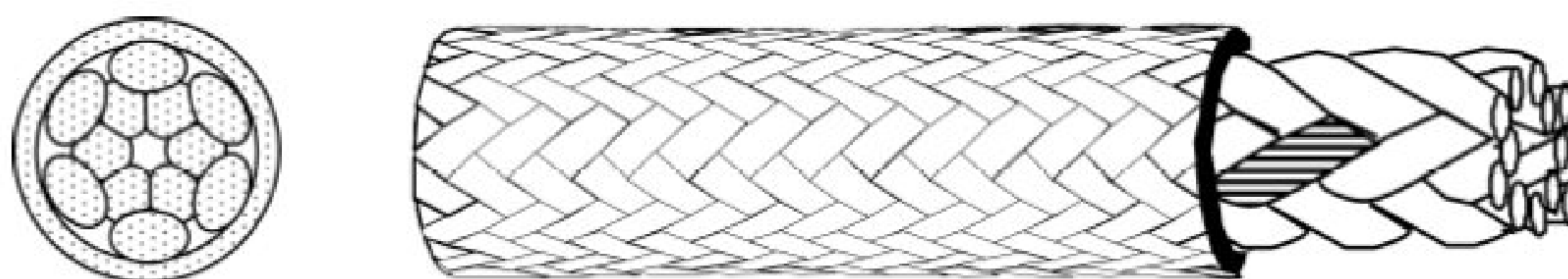
а) Канат с одним сердечником в оболочке
