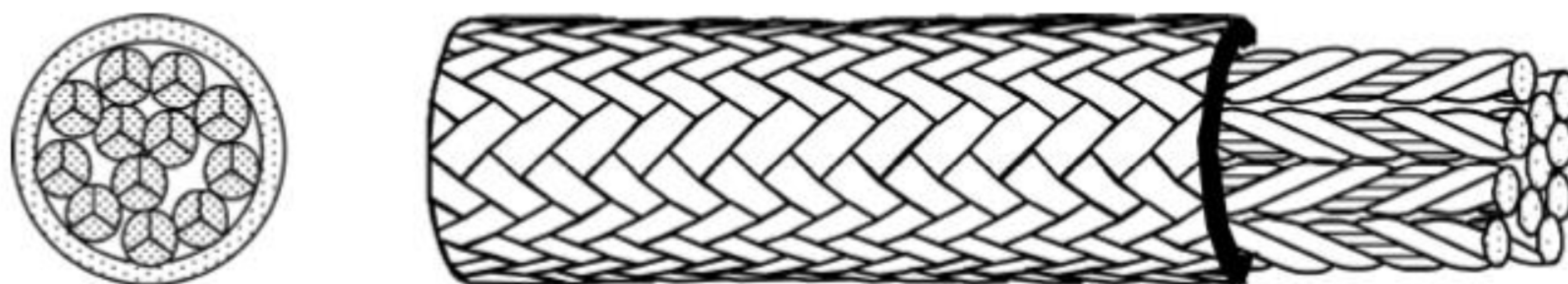
б) Канат с несколькими сердечниками: 3-рядные сердечники
