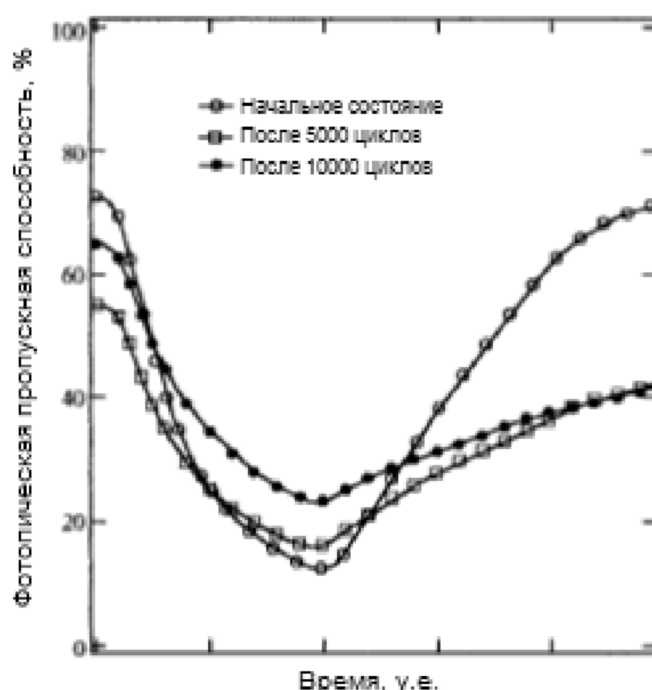
Рисунок 5 — Фотопропускная способность как функция времени, измеренного на различных этапах циклических испытаний типового окна с ЭХП
