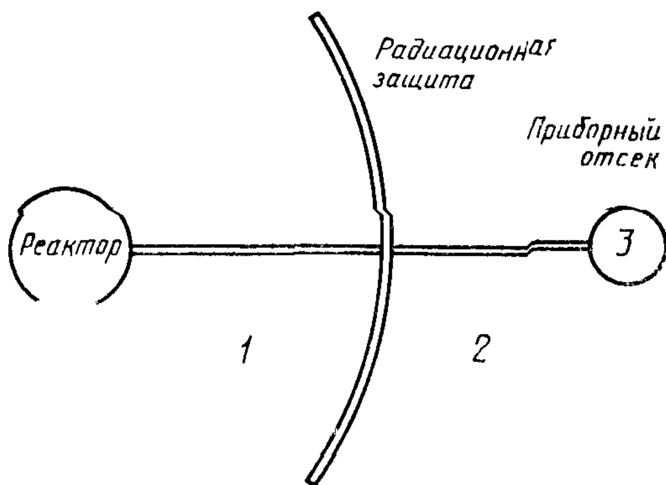
Рисунок 1 — Схема космического аппарата с бортовым ядерным реактором
