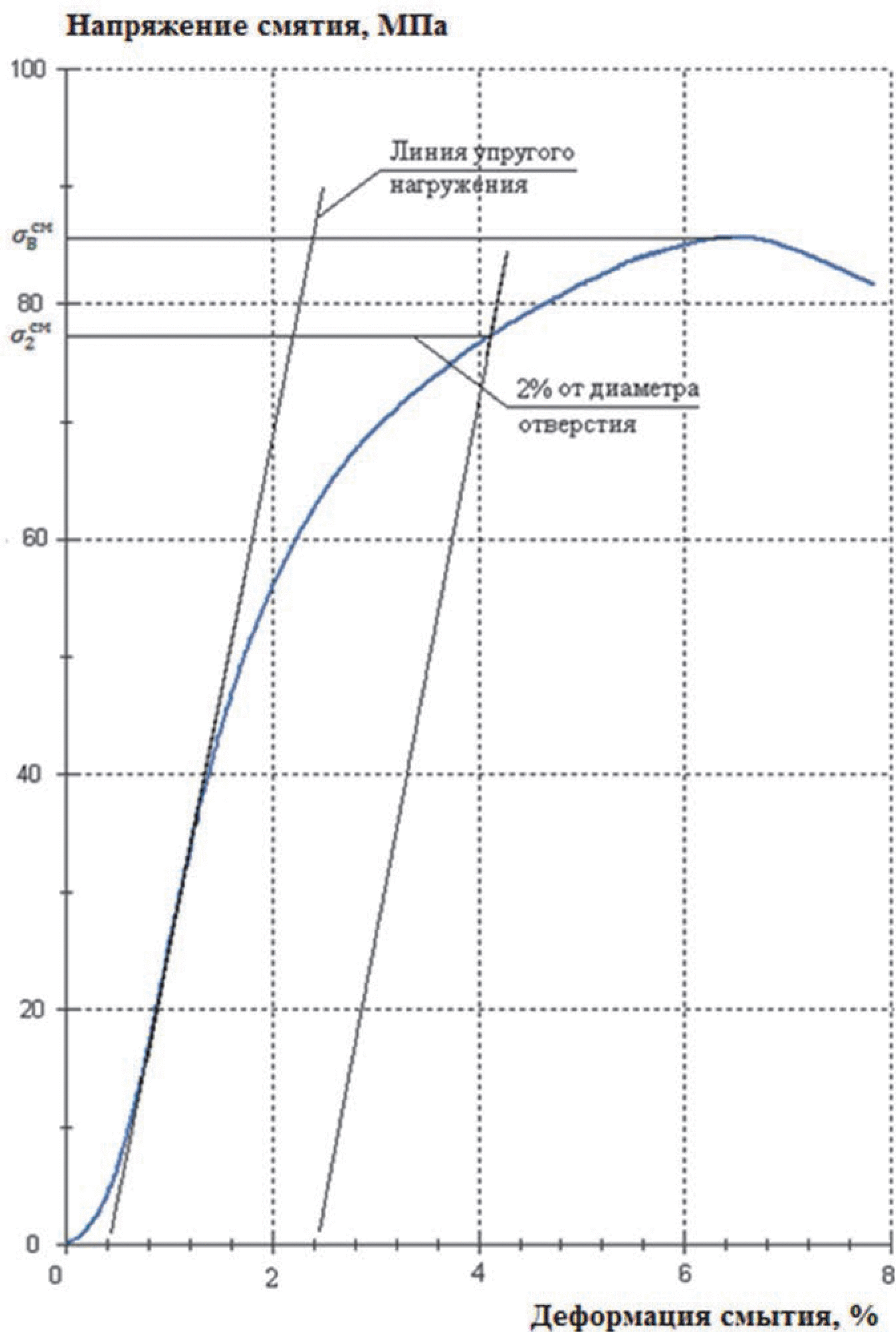
Рисунок 6 — Диаграмма смятия
