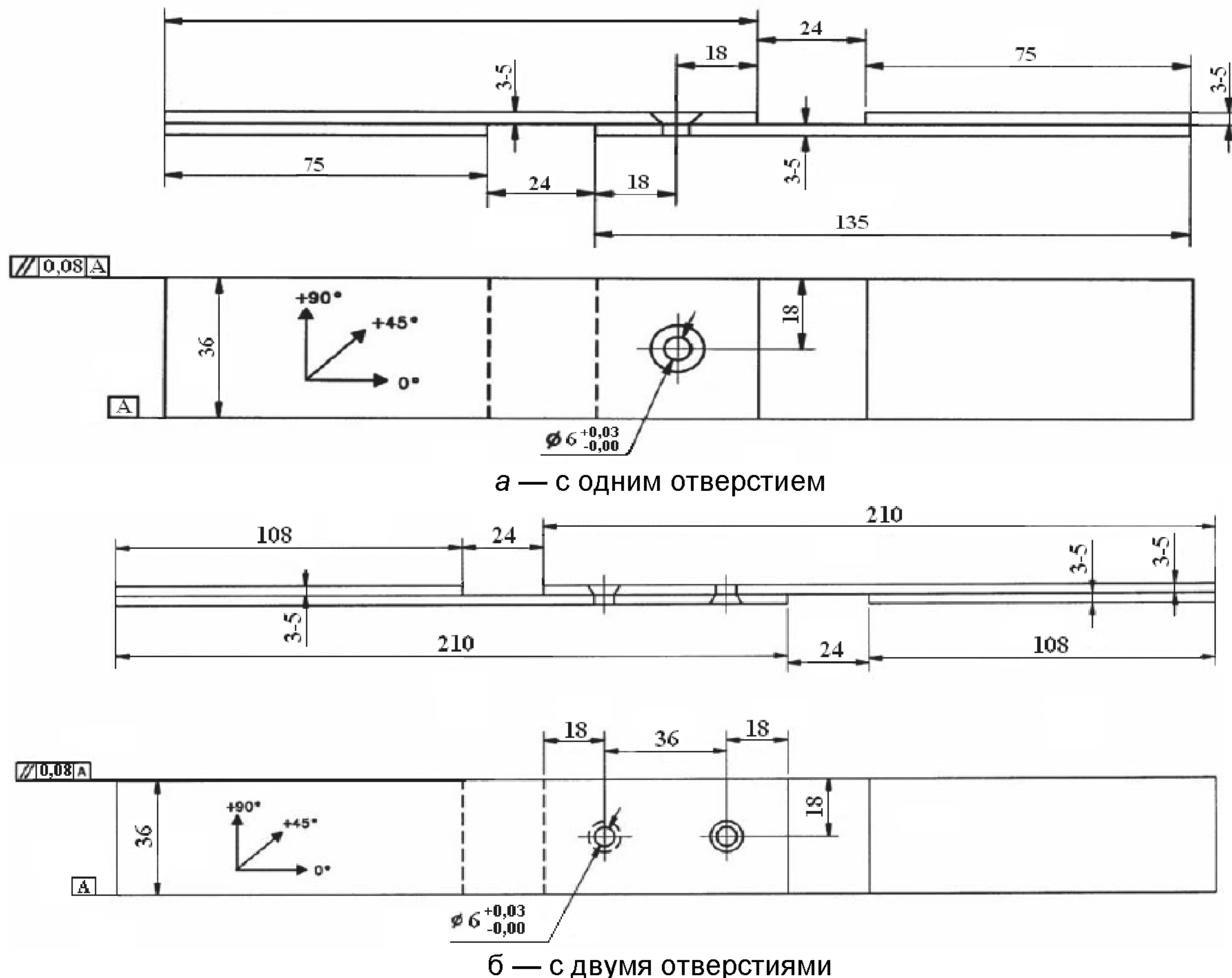
Рисунок 4 — Составной образец ПК
