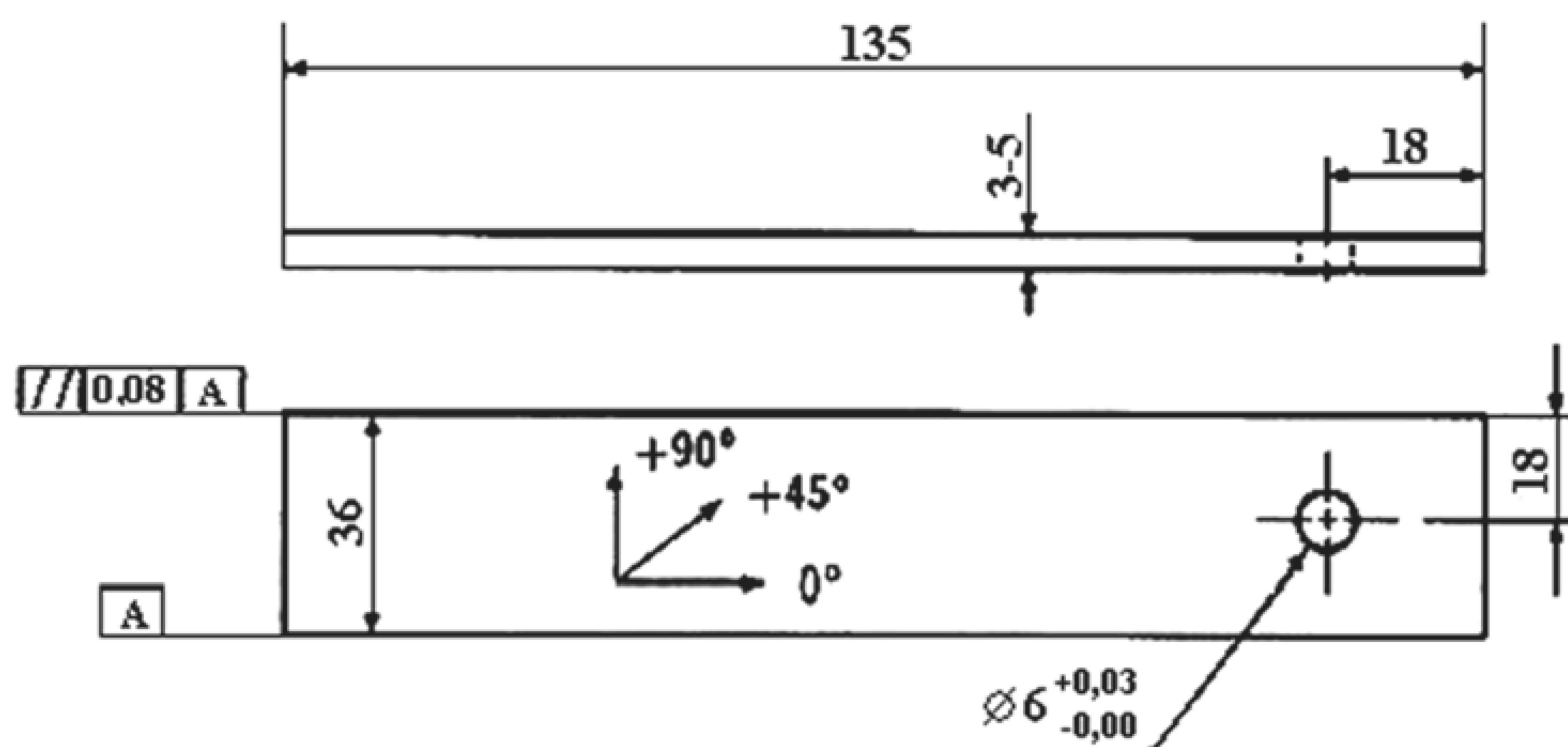
Рисунок 2 — Образец ПК с одним отверстием
