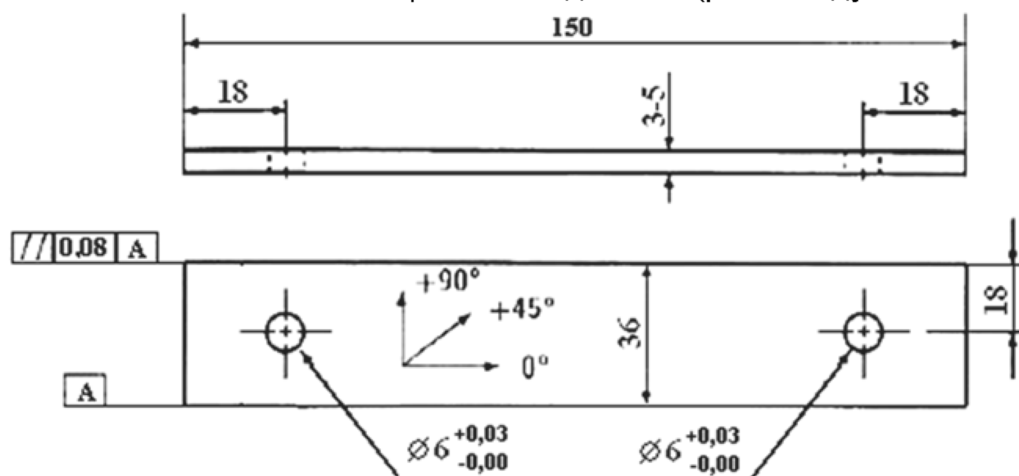
Рисунок 3 — Образец ПК с двумя отверстиями
