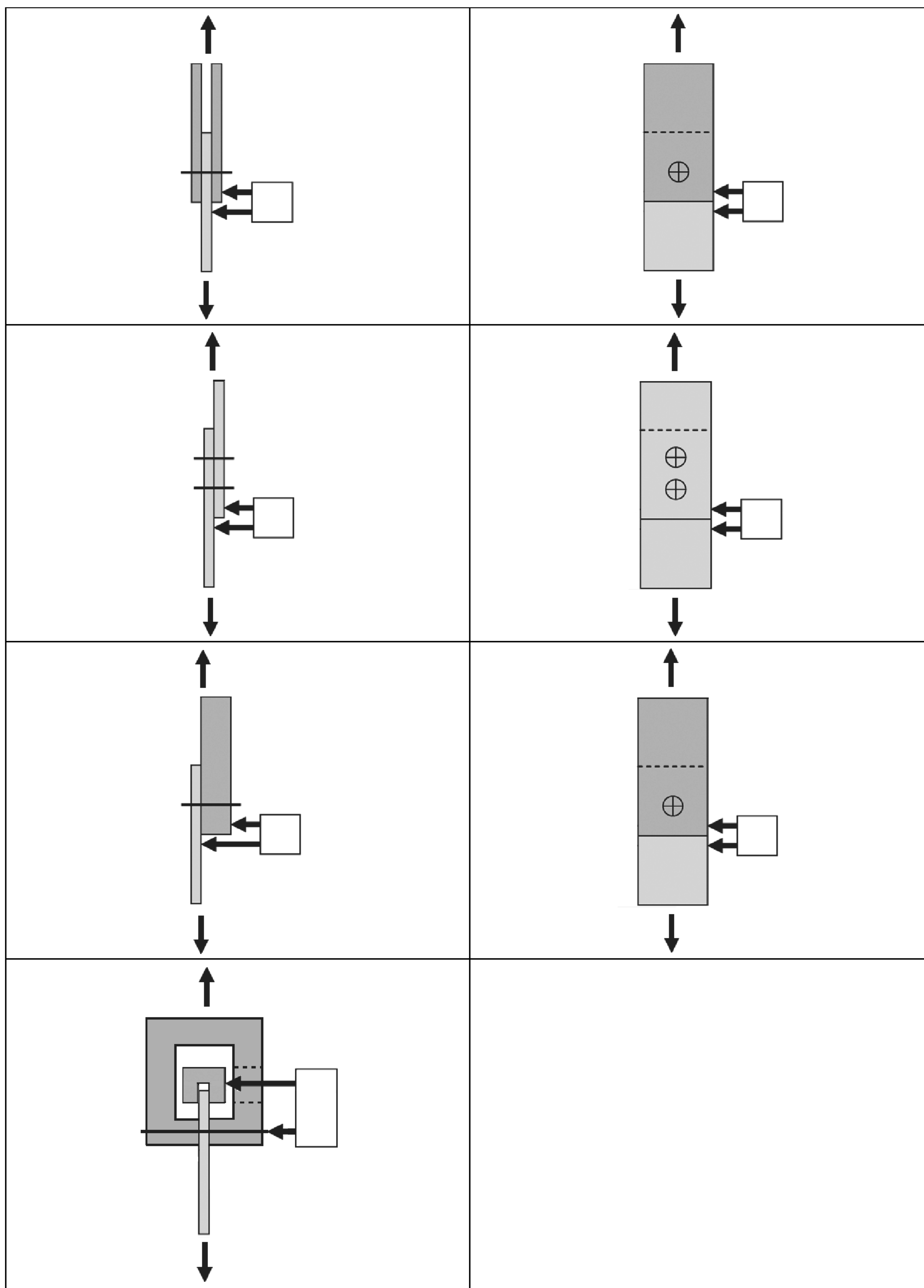
Рисунок 1 — Установка датчика деформации
