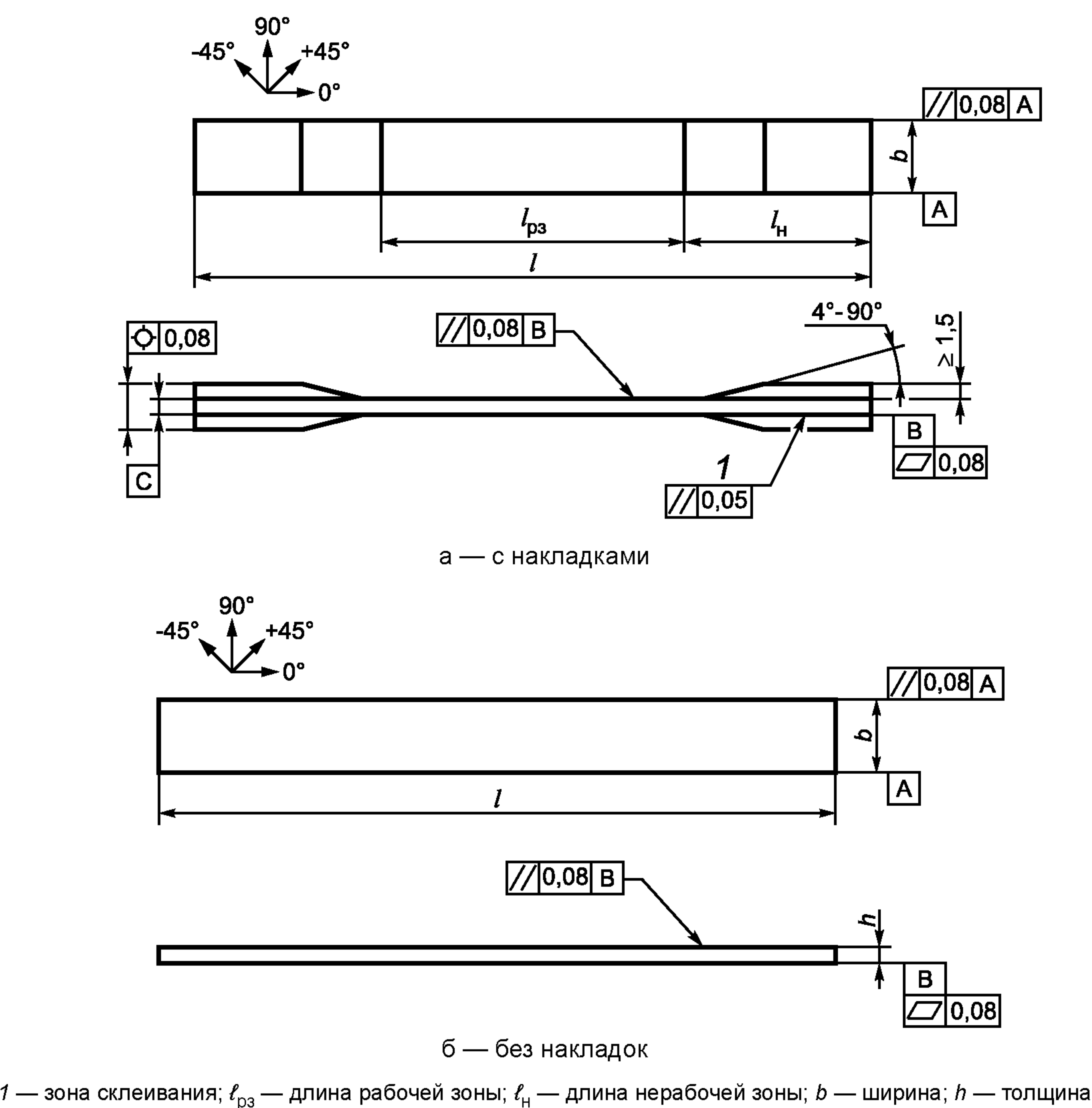
Рисунок 2 — Образец из композитного материала для испытаний на растяжение
