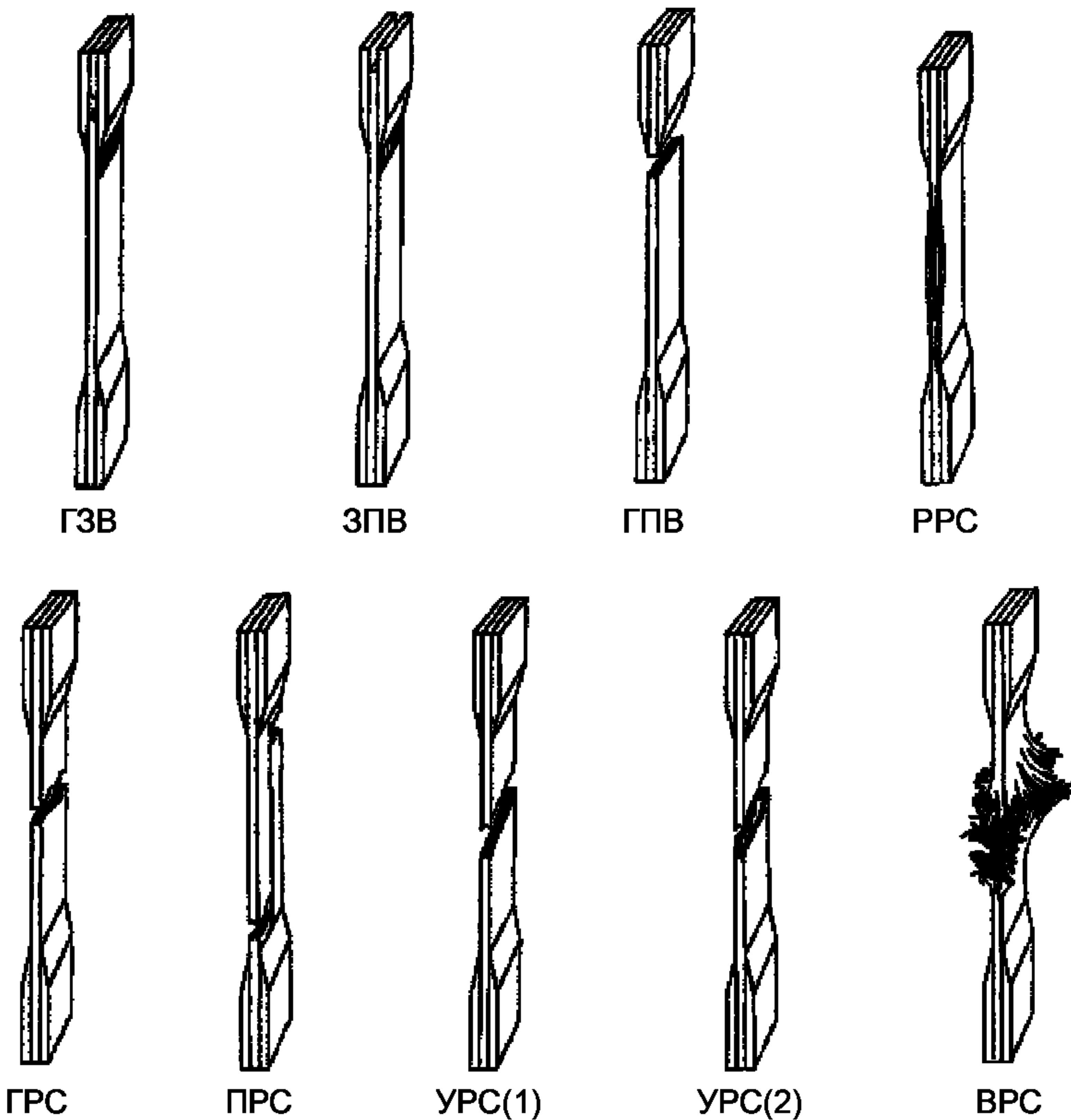
Рисунок 4 — Примеры обозначения типовых разрушений
