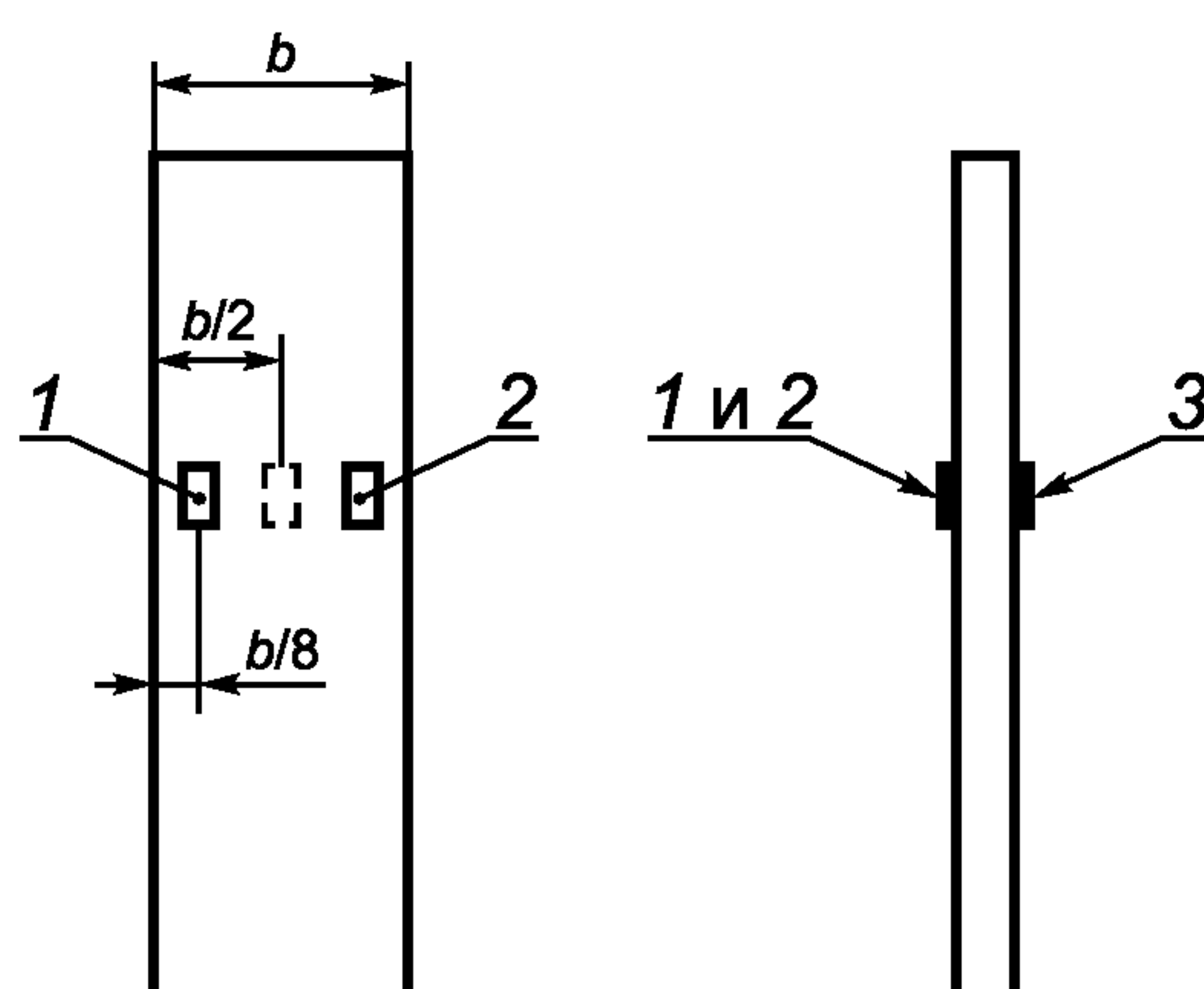
b — ширина образца; 1, 2, 3 — датчики
