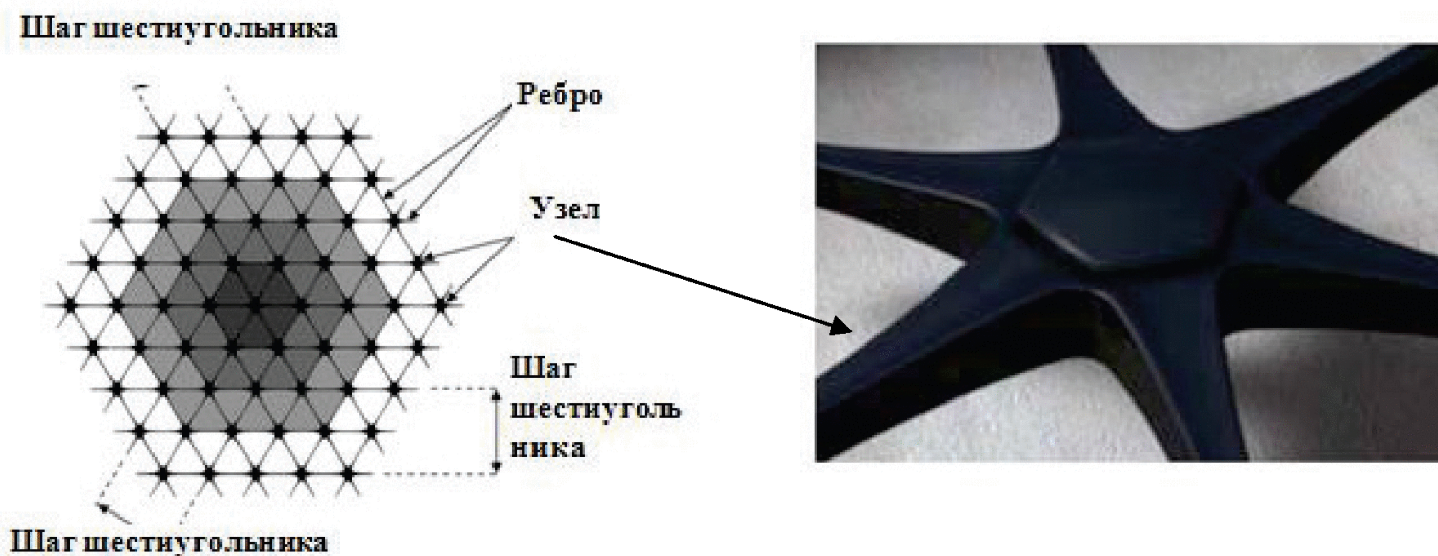
Рисунок 1 — Схематическое изображение георешетки и ее узел
