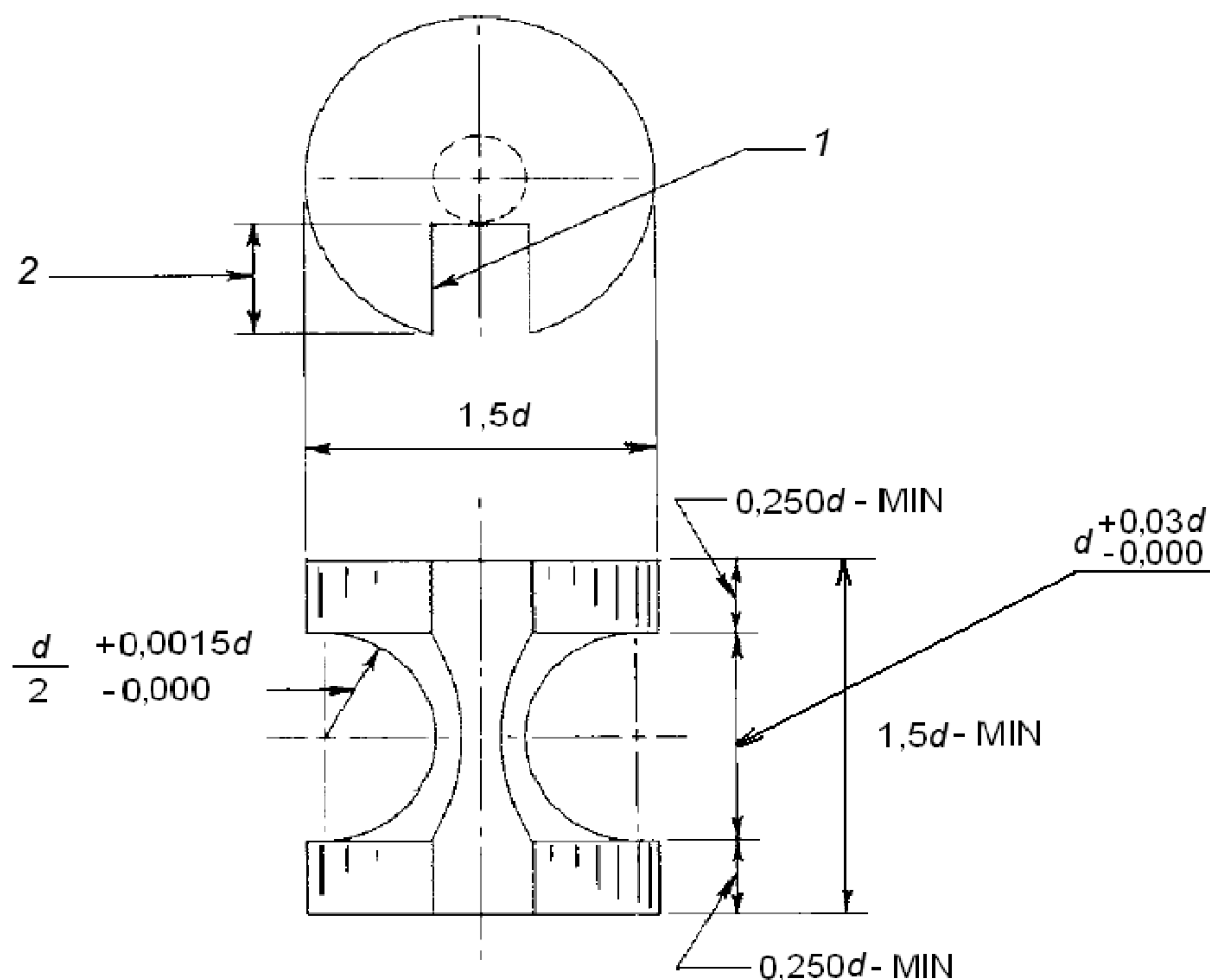
Рисунок 1 – Геометрические размеры пуансона и опор
