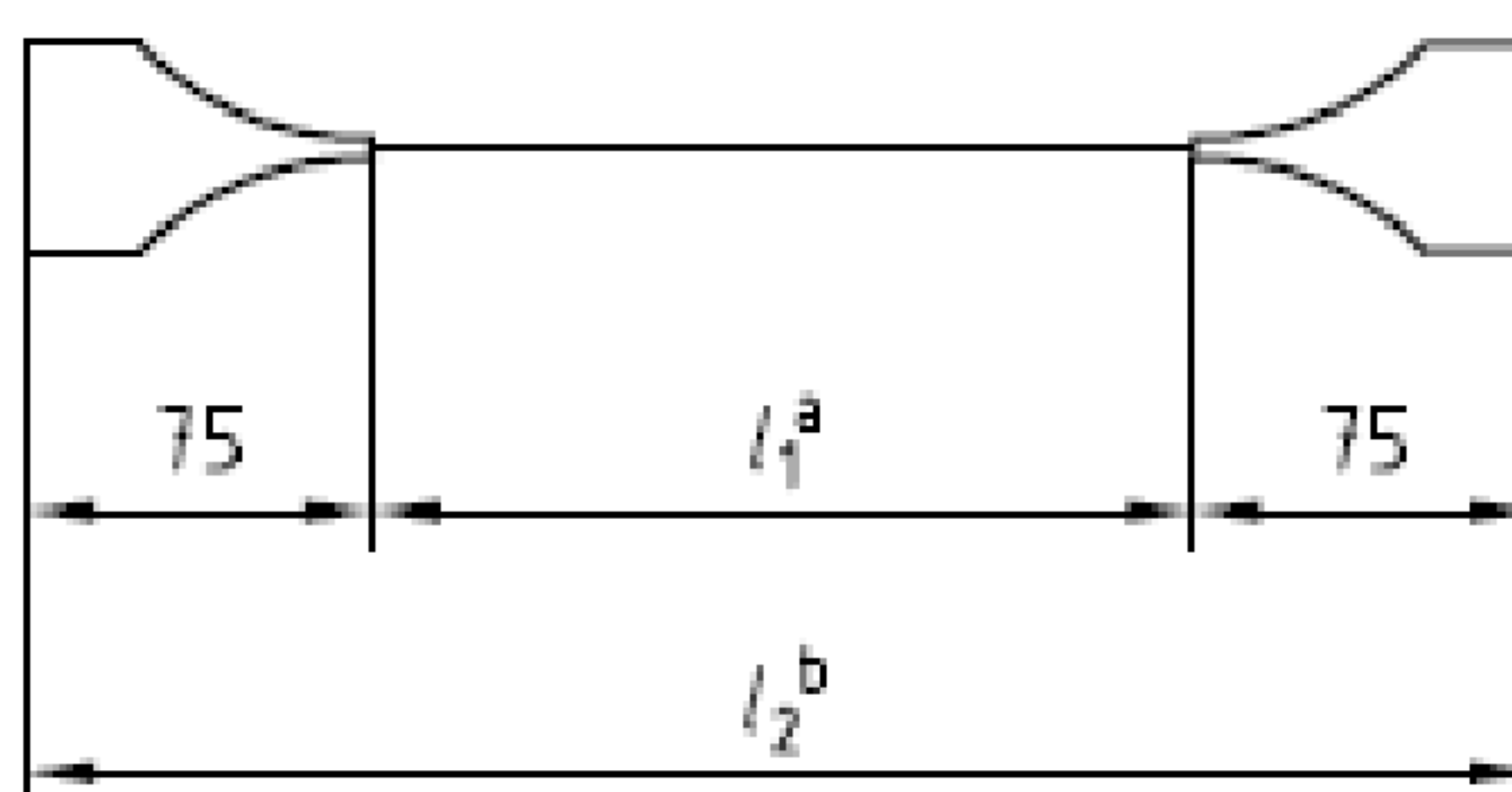
Рисунок С.1 — Термопластмассовые петли
