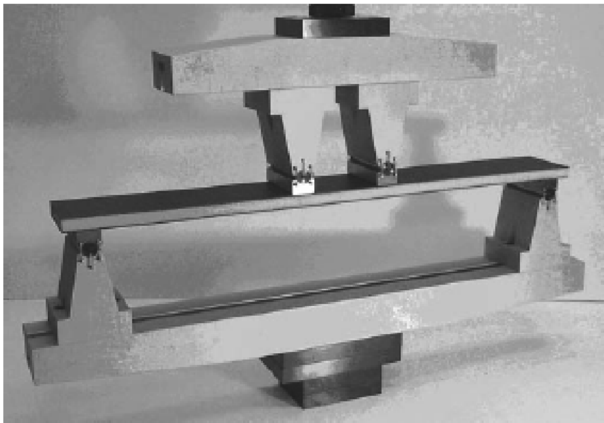
Рисунок 3 — Стандартная схема нагружения в четырех точках
