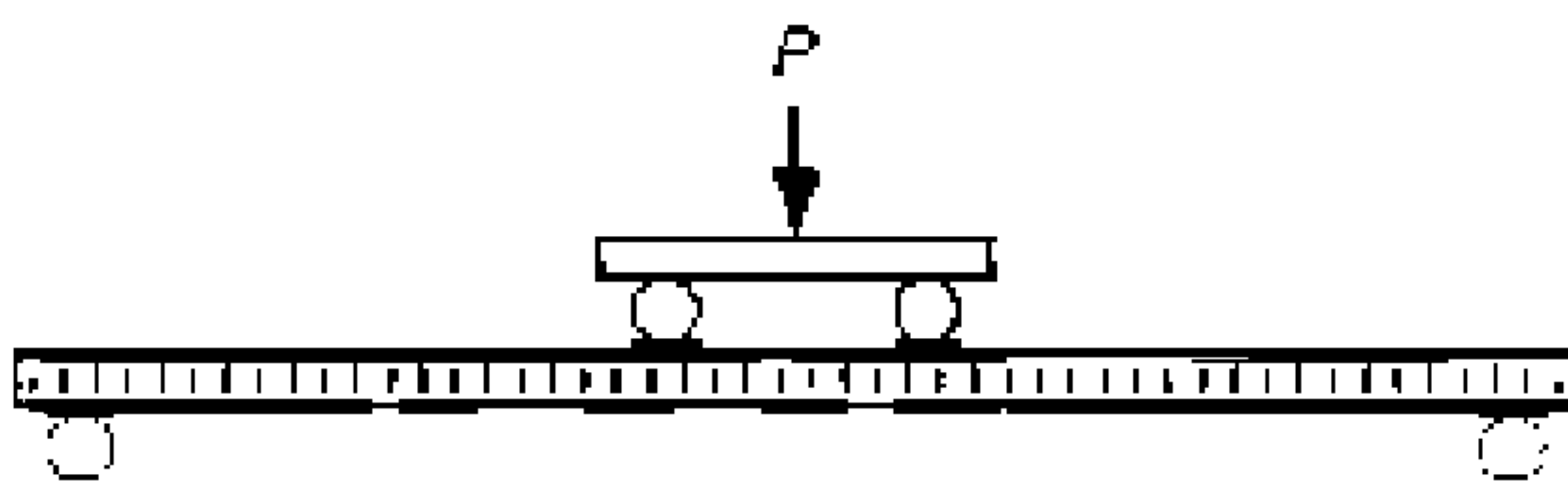
Рисунок 1 — Испытываемый образец и приспособление для проведения испытания
