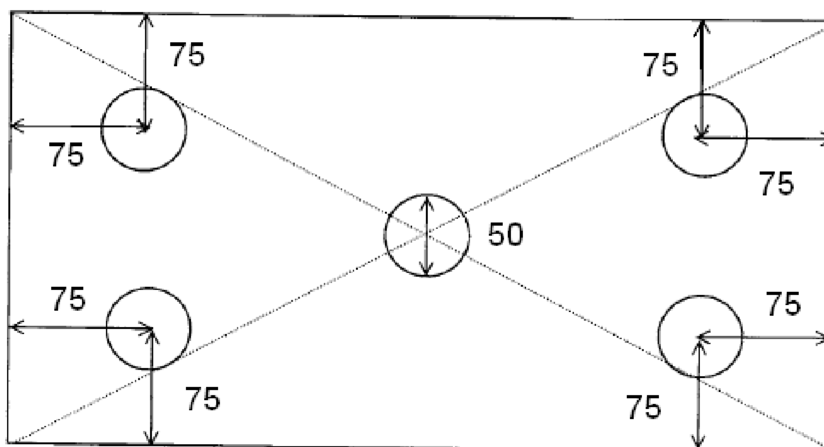
Рисунок 1 — Схема расположения контрольных точек
