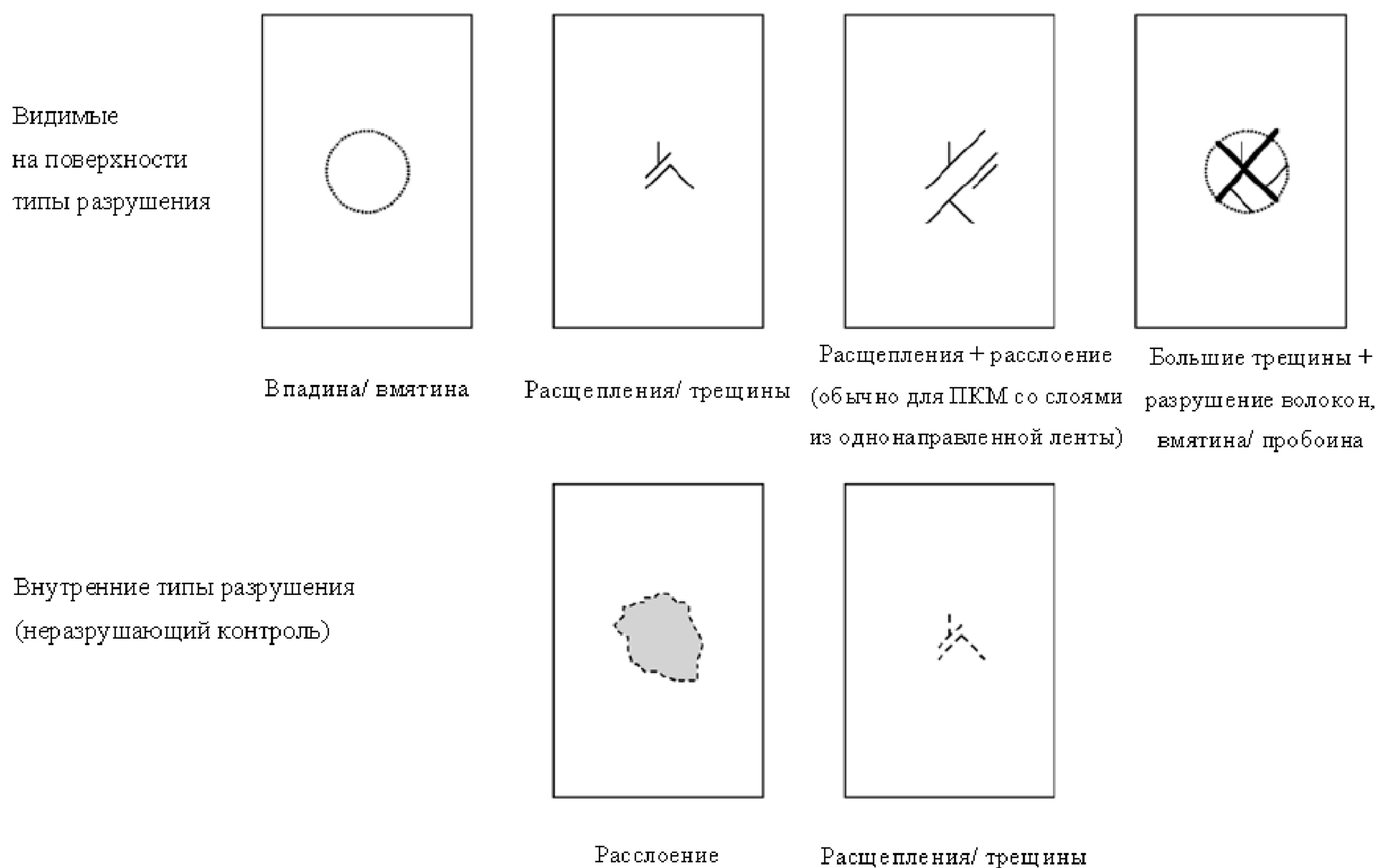
Рисунок 9 — Типовые повреждения в результате удара
