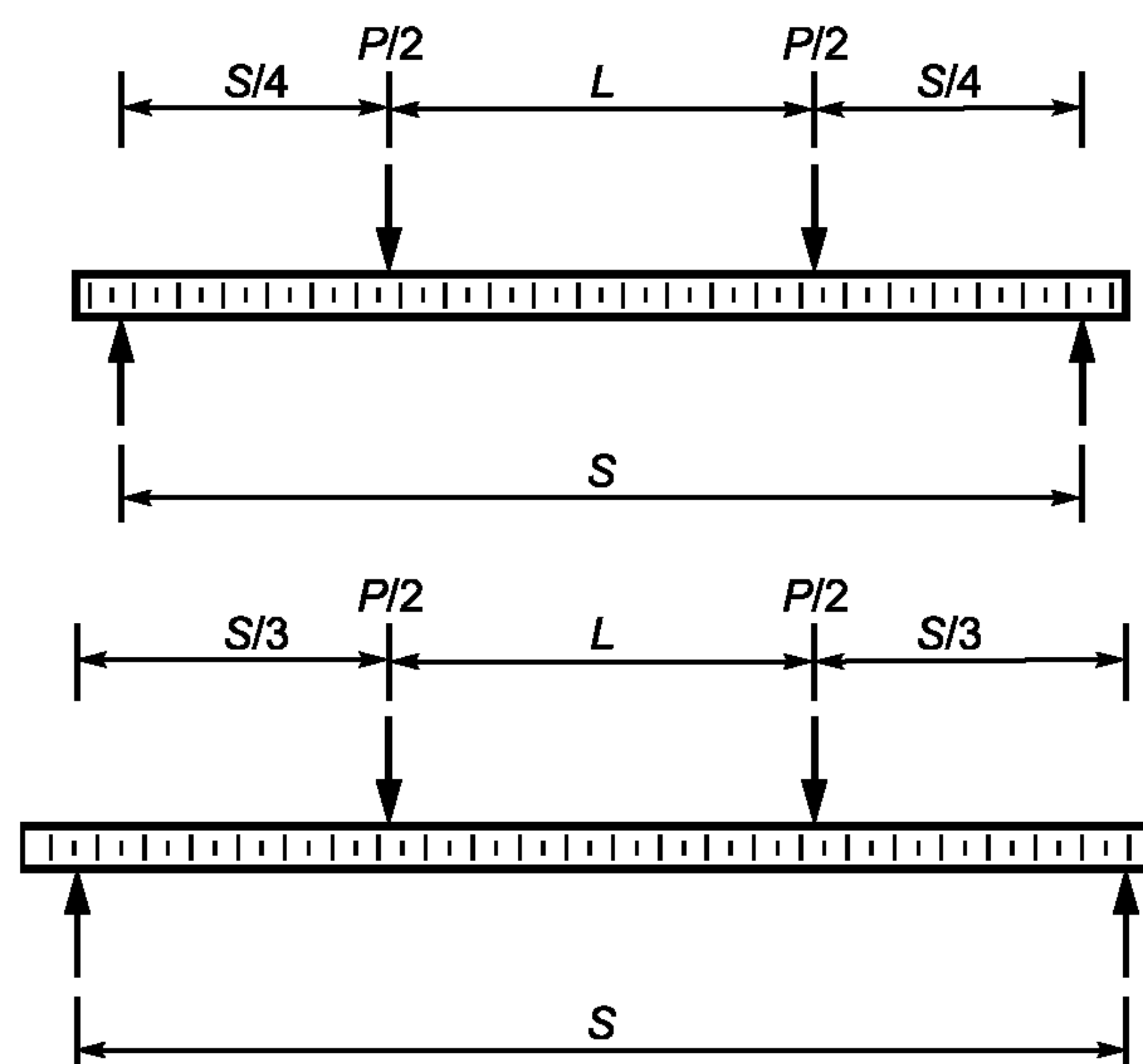
(с) четырехточечное нагружение (С393/С393М нестандартная схема)
