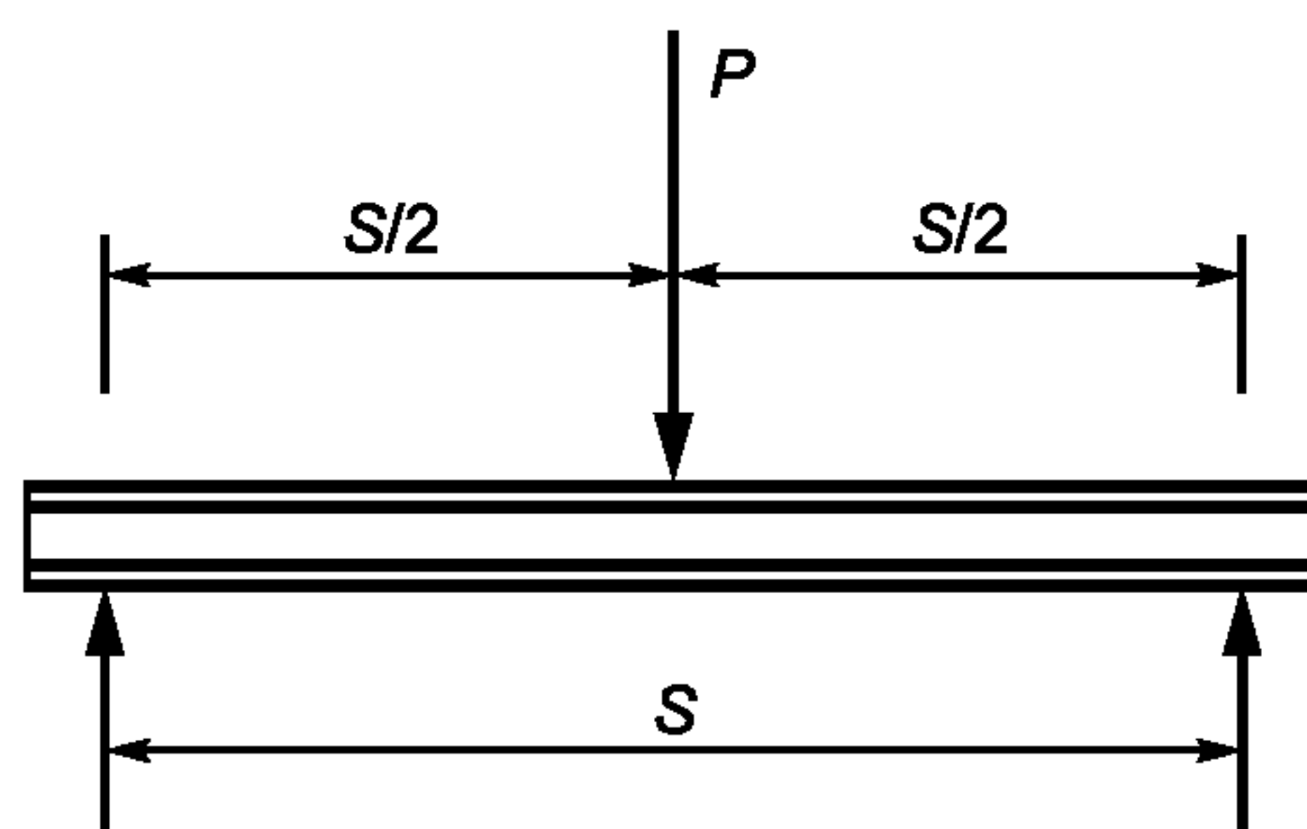
(а) трехточечное нагружение (С393/С393М стандартная схема)
