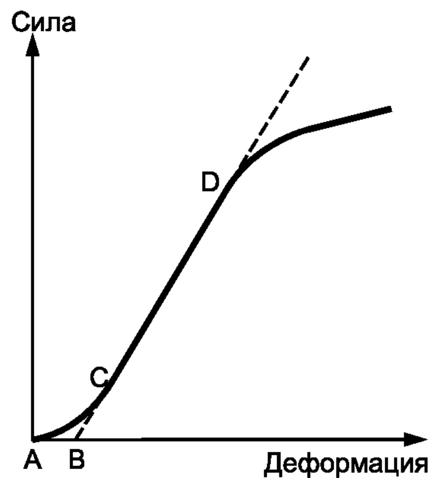
Рисунок А.1 — График зависимости силы от деформации
