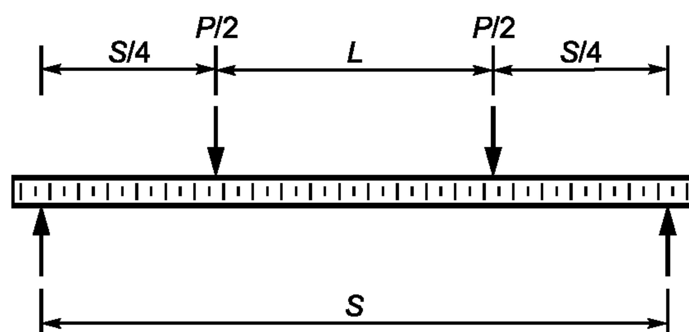
(b) четырехточечное нагружение (D7249/D7249ML стандартная схема для длинной балки)
