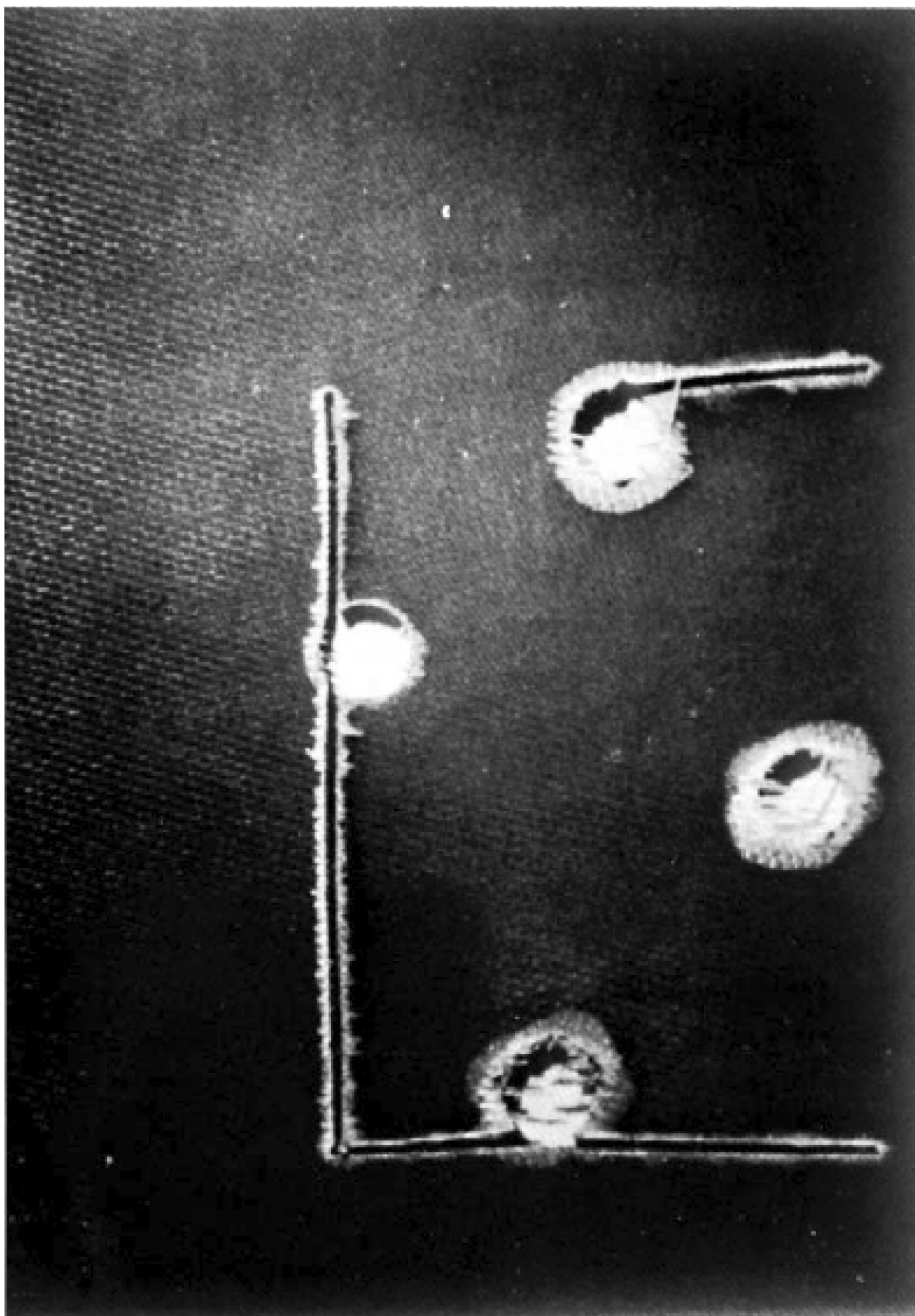
Рисунок А.3 — Расслаивание вследствие неправильной механической обработки
