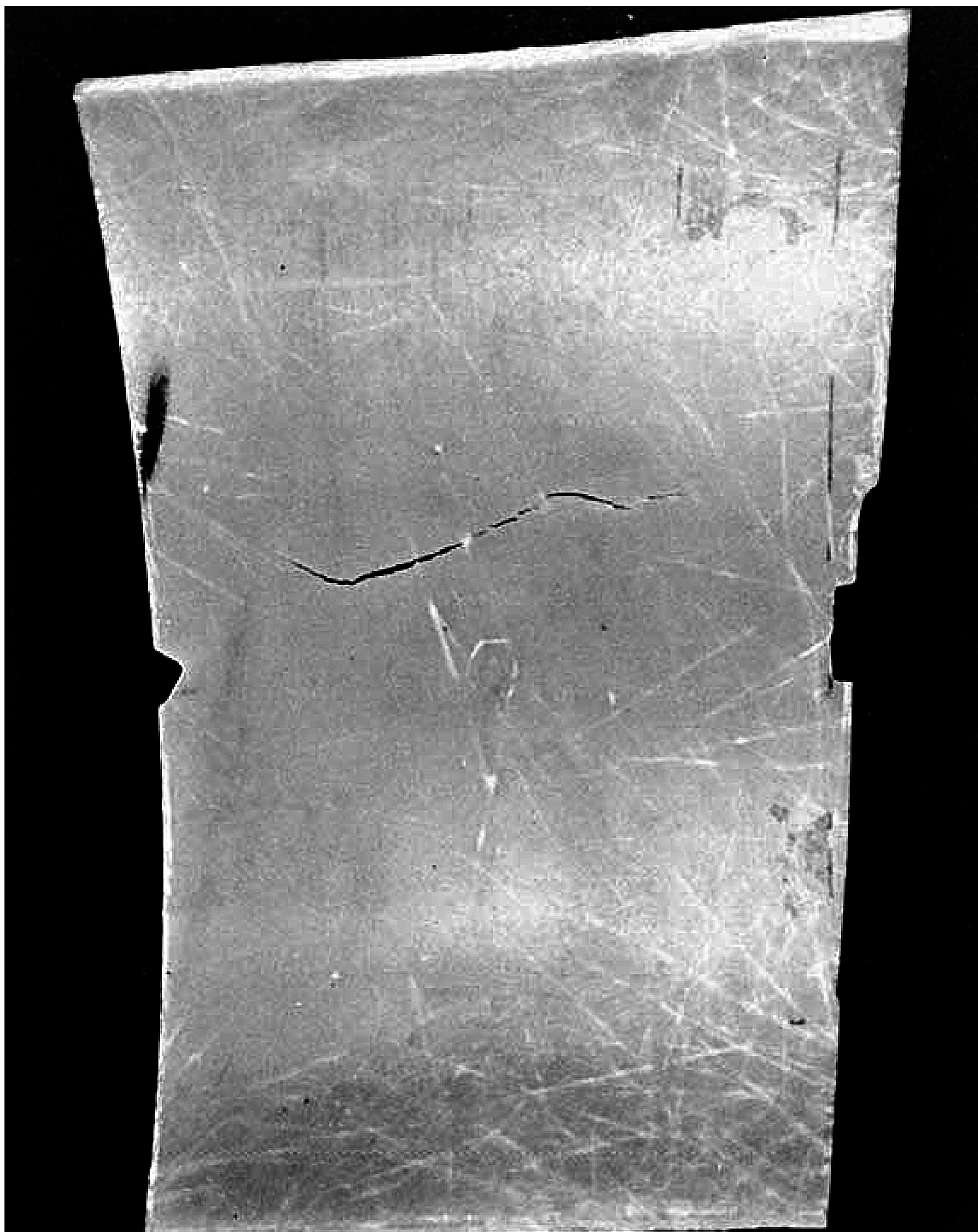
Рисунок А.15 — Трещина с избыточной смолой
