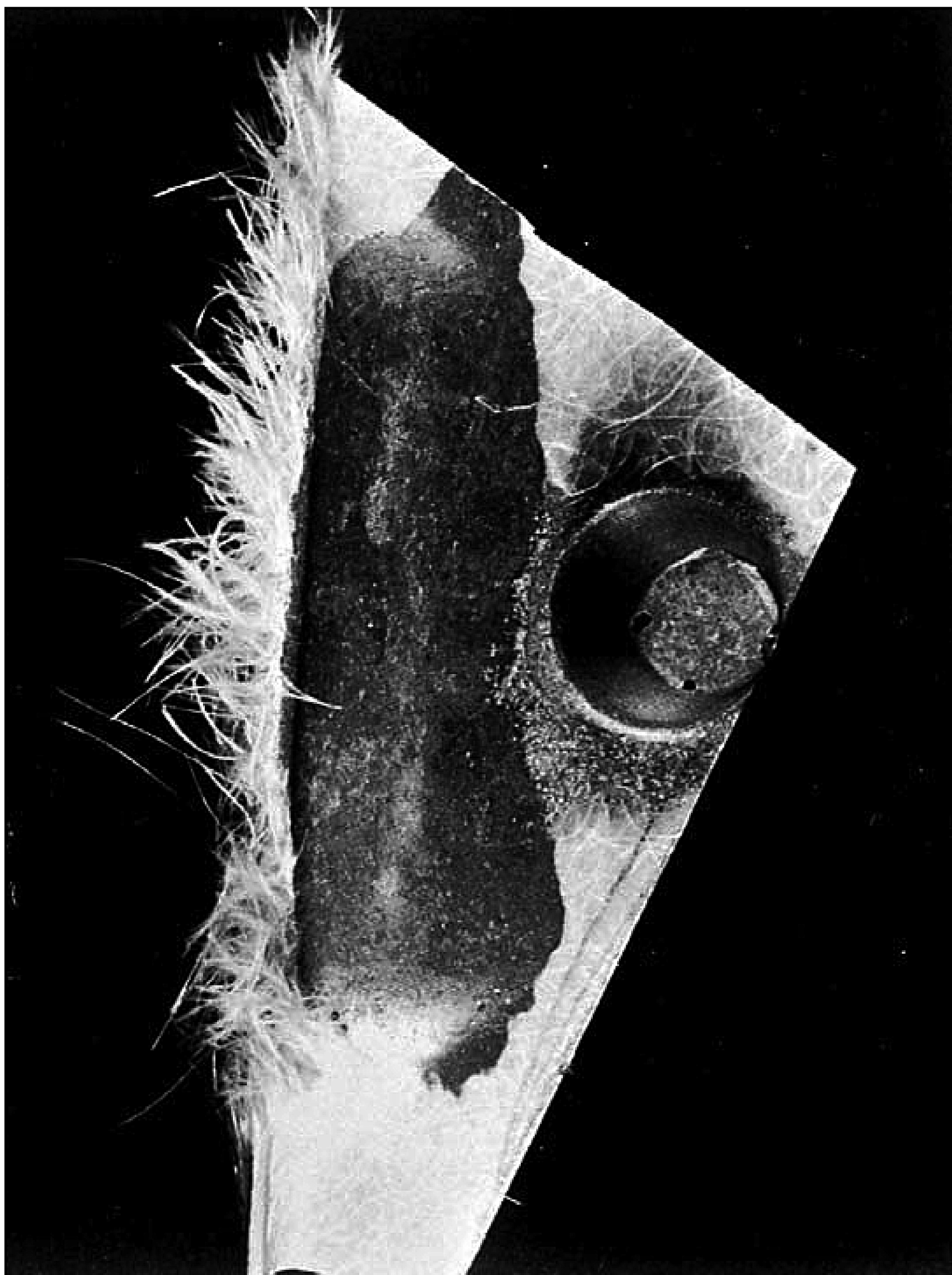
Рисунок А.11 — Непропитанный участок
