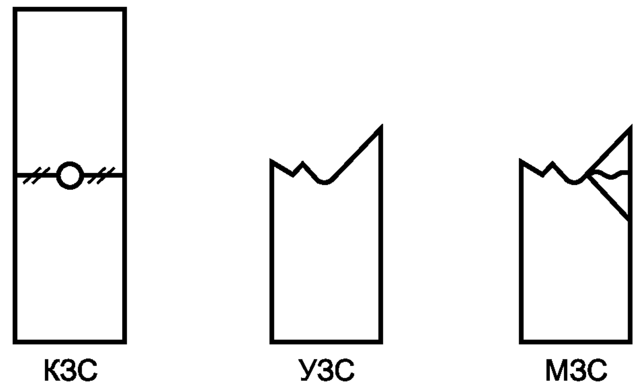
Рисунок 2 — Примеры допустимых типов разрушения
