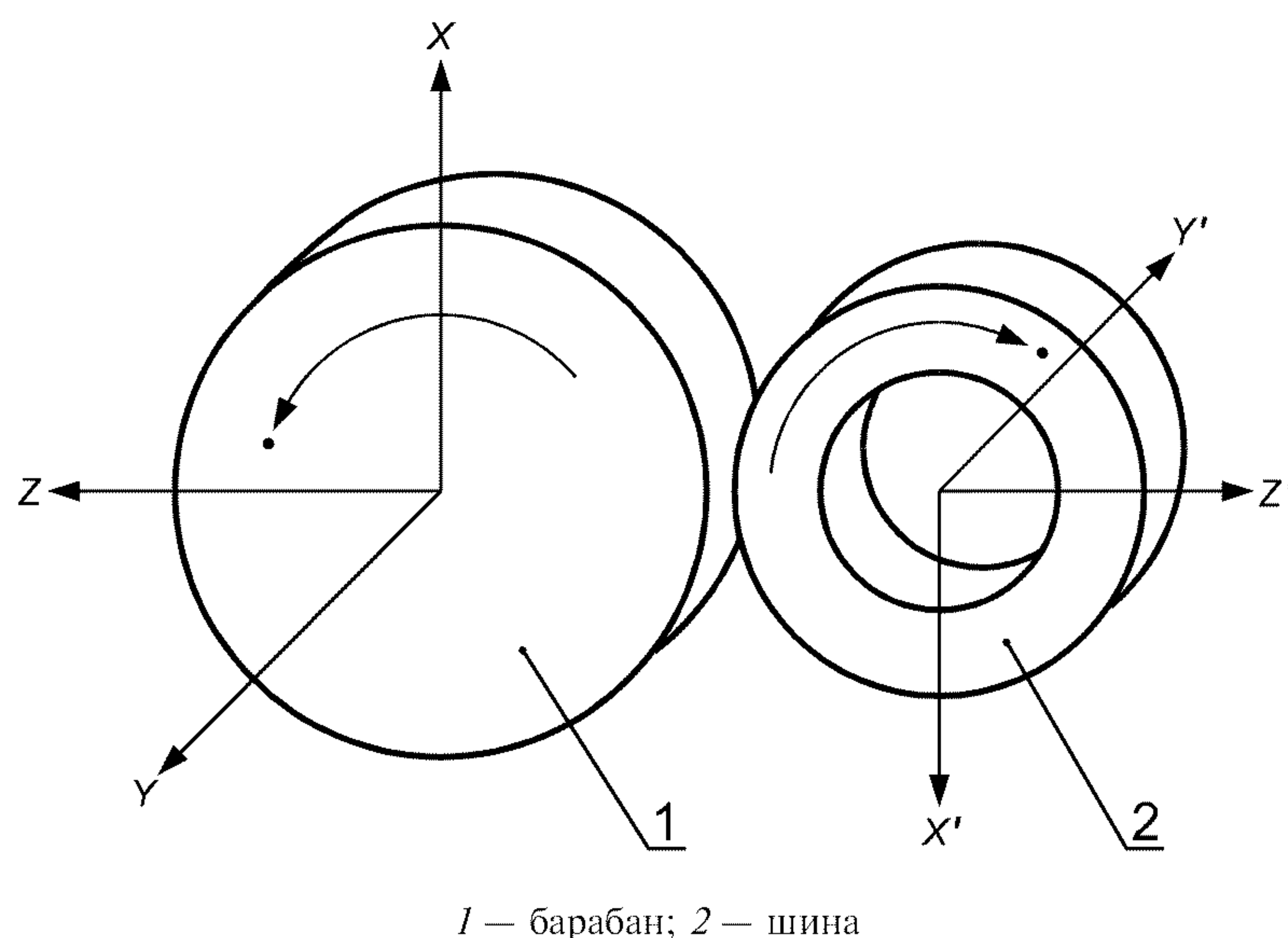
Рисунок 1 — Система базисных осей для сил
