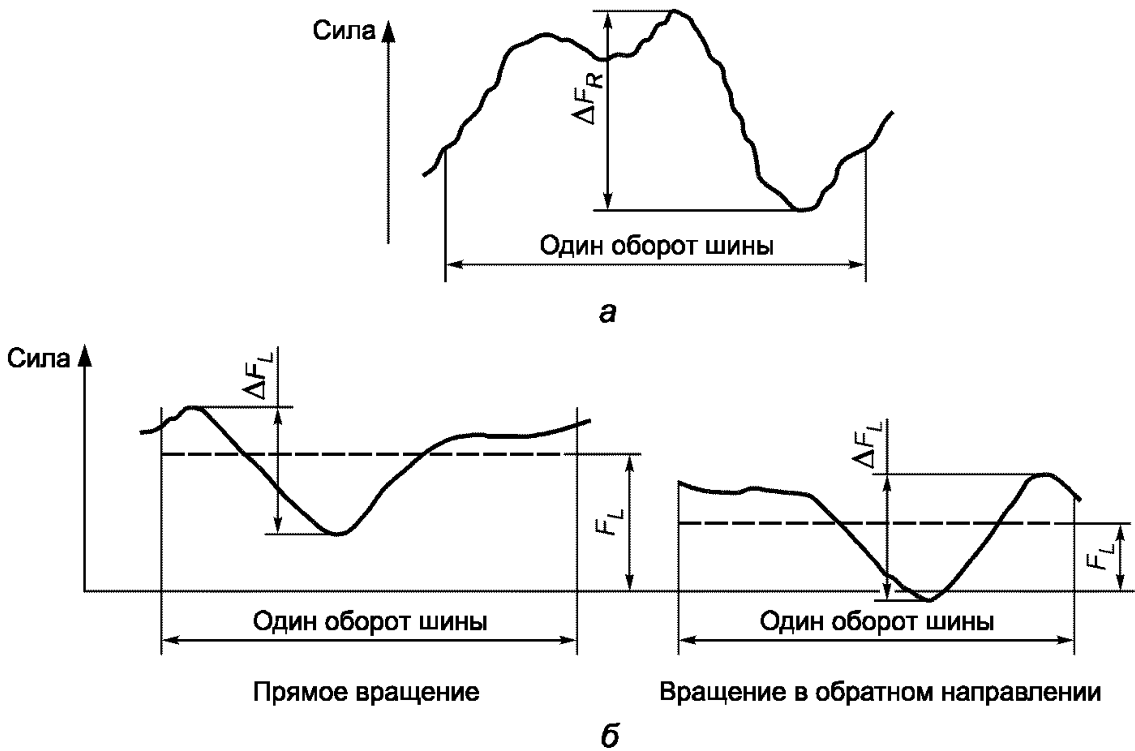
a — радиальная сила; b — боковая сила
