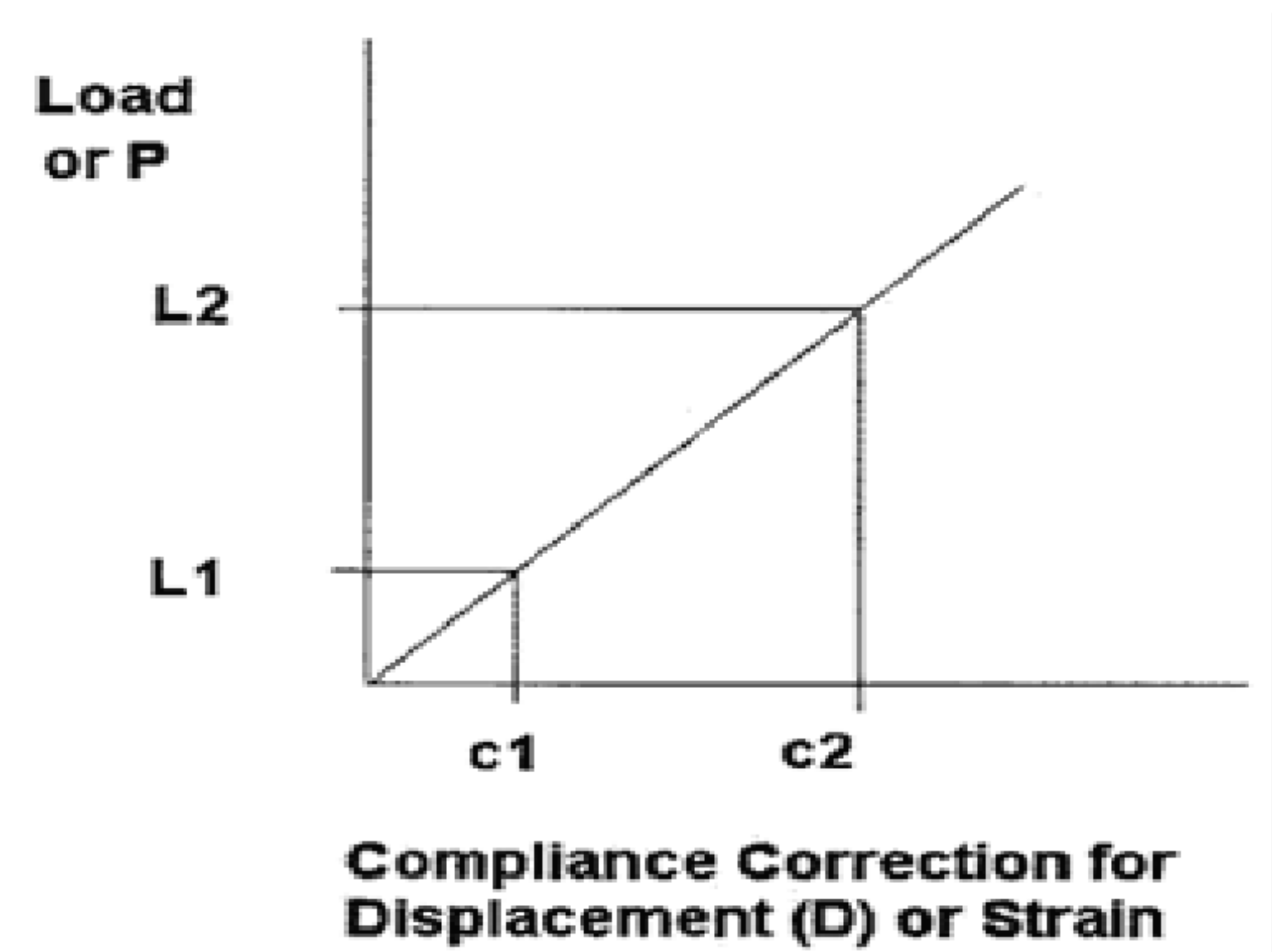
Рисунок X1.2 — Кривая соответствия для стального стержня
