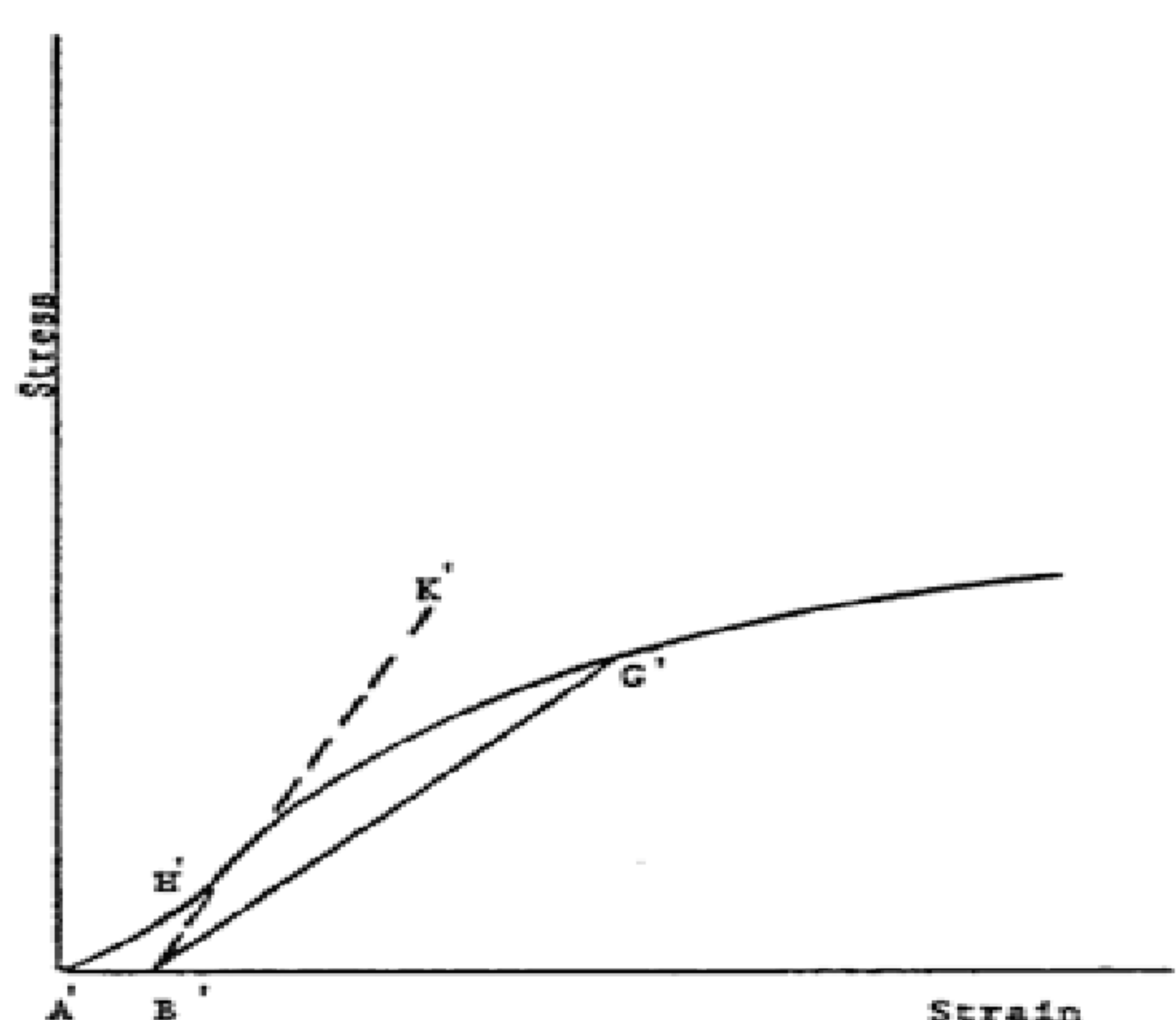
Рисунок A1.2 — Материал с отсутствием линейно-упругой области
