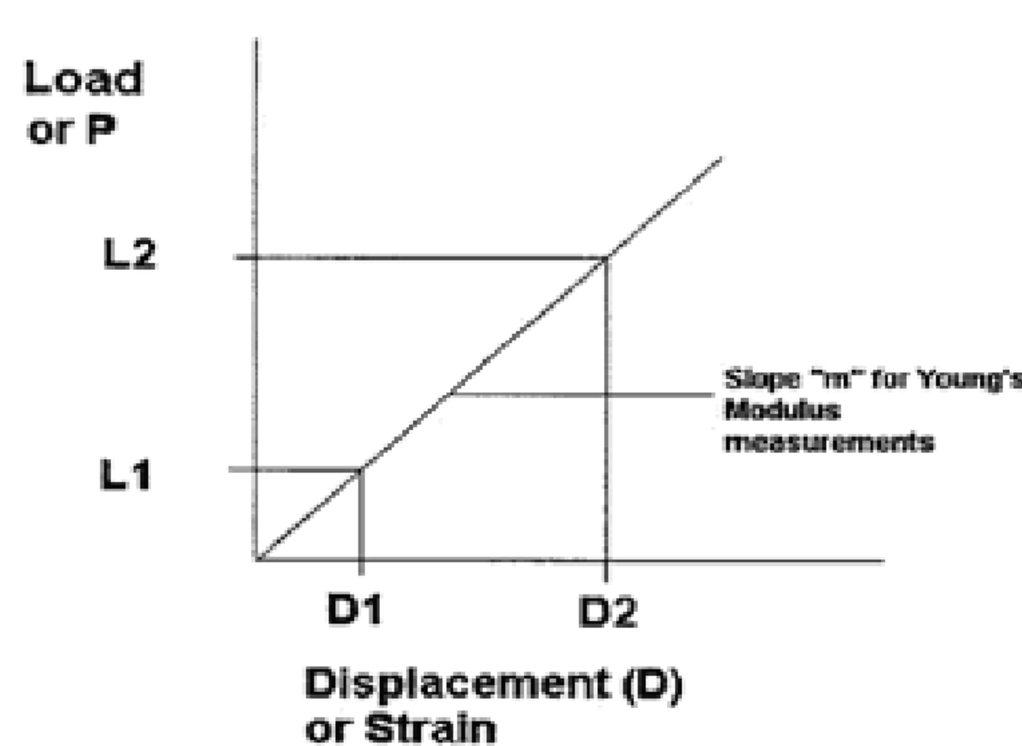
Рисунок X1.1 — Пример кривой модуля для материала
