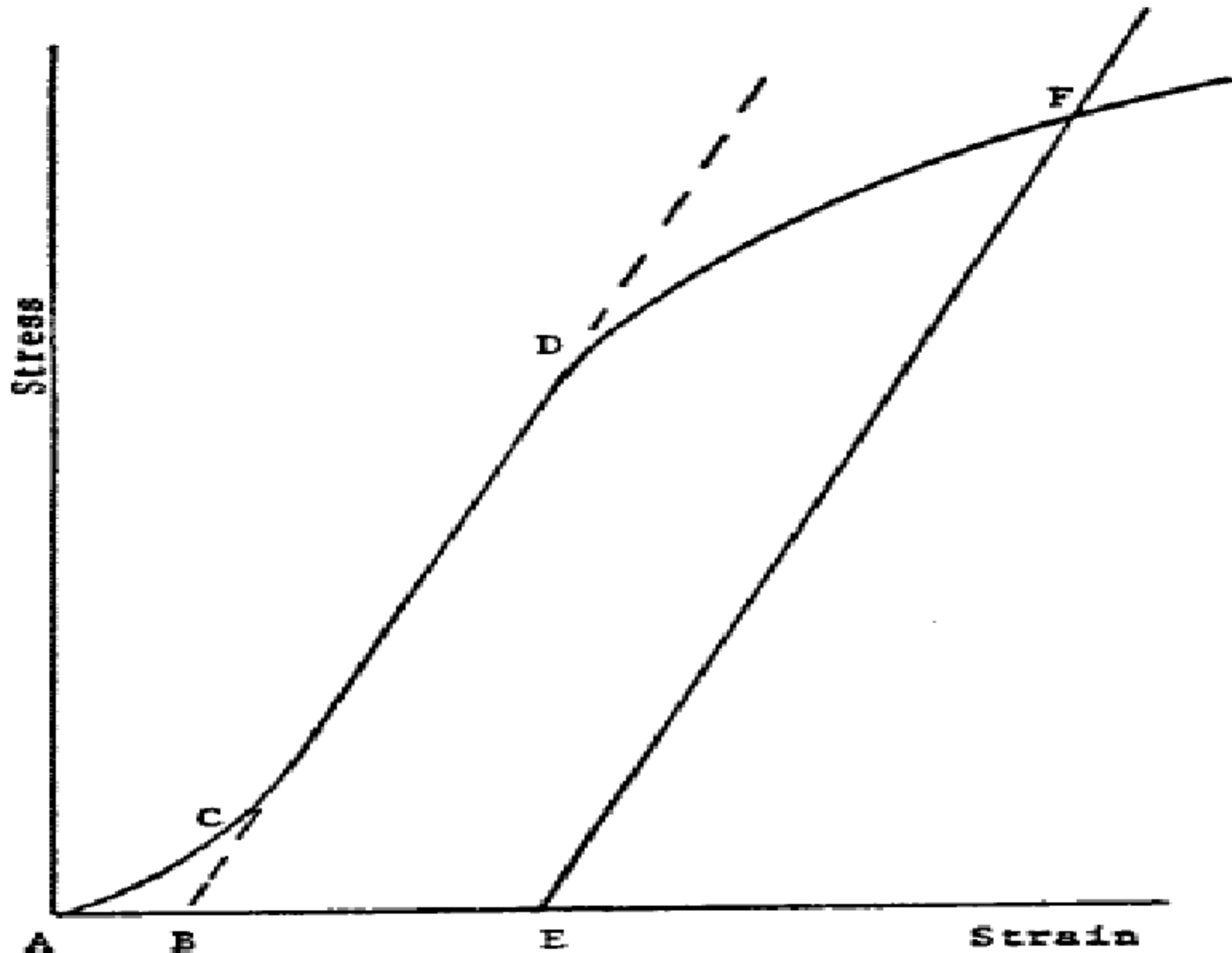
Рисунок А1.1 — Материал с линейно-упругой областью
